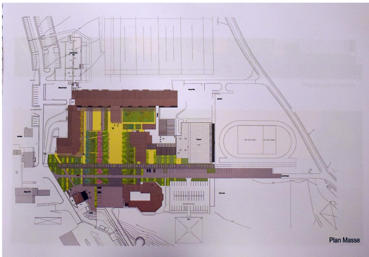
Plan masse (A Région Auvergne-Rhône-Alpes site de Clermont-Ferrand, 806 WR 8)
