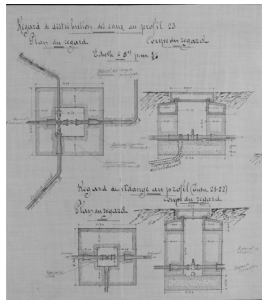
Plan et coupe d'un regard de distribution des eaux au profil 23. Plan et coupe d'un regard de vidange des eaux au profil 21-22, par [Bertrand architecte, février 1904]. Phot. Alain Franchella IVR82_19972600535X
