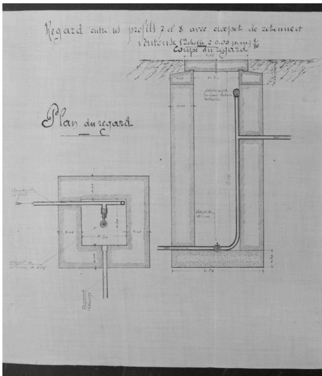
Plan et coupe d'un regard entre les profils 7 et 8, par [Bertrand architecte, février 1904].
