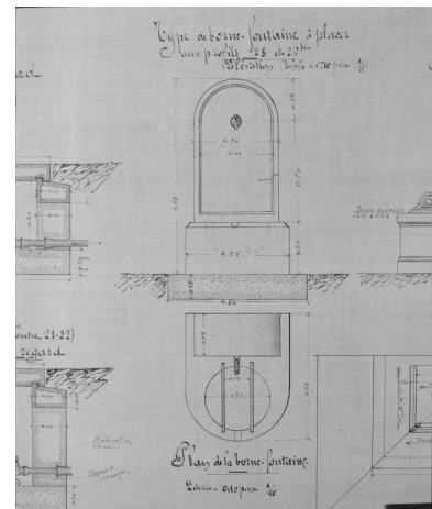
Elévation et plan d'une borne-fontaine, par [Bertrand architecte, février 1904]. Phot. Alain Franchella IVR82_19972600534X
