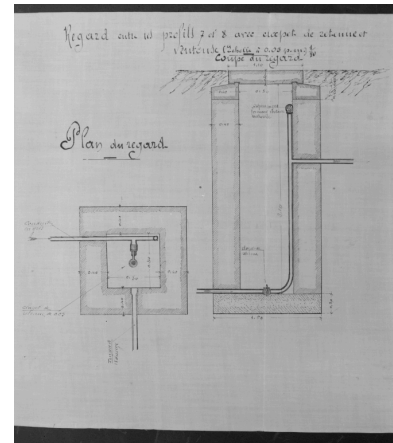
Plan et coupe d'un regard entre les profils 7 et 8, par [Bertrand architecte, février 1904]. Phot. Alain Franchella IVR82_19972600537X
