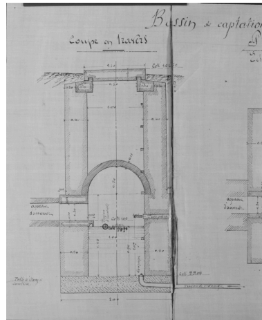
Coupe en travers d'un réservoir d'eau alimentant la commune, par [Bertrand architecte, février 1904]. Phot. Alain Franchella IVR82_19972600526X
