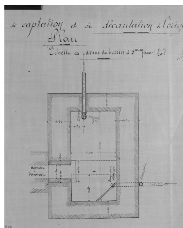
Plan d'un réservoir d'eau alimentant la commune, par [Bertrand architecte, février 1904]. Phot. Alain Franchella IVR82_19972600525X
