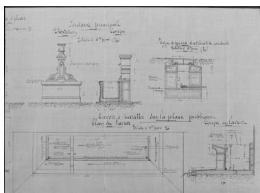
Elévation et coupe de la fontaine principale ; coupe d'un regard ; plan et coupe du lavoir à installer sur la place publique, par [Bertrand architecte, février 1904]. Phot. Alain Franchella IVR82_19972600533X
