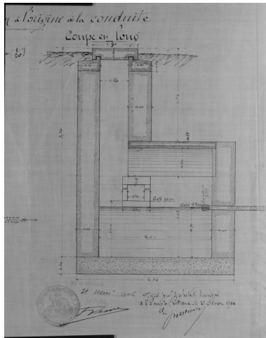
Coupe en long d'un réservoir d'eau alimentant la commune, par [Bertrand architecte, février 1904]. Phot. Alain Franchella IVR82_19972600524X
