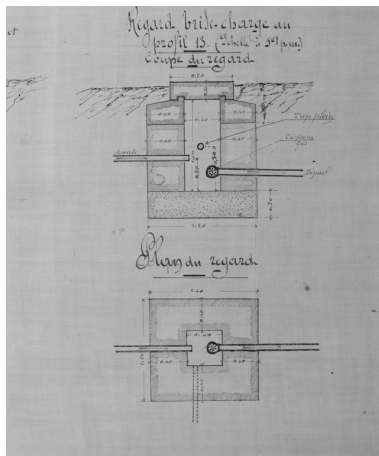
Plan et coupe d'un regard brise-charge au profil 13, par [Bertrand architecte, février 1904]. Phot. Alain Franchella IVR82_19972600536X
