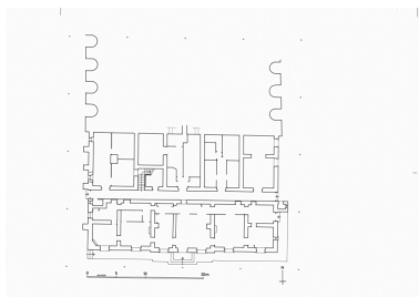
Plan de l'étage de soubassement. Dessin Inventaire P.Cherblanc, 1997, d'après plan anonyme, 1969. Phot. Jean-Marie Refflé IVR82_19970100013P
