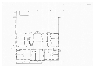
Plan du rez-de-chaussée surélevé. Dessin Inventaire P.Cherblanc, 1997, d'après plan anonyme, 1969. Phot. Jean-Marie Refflé IVR82_19970100014P
