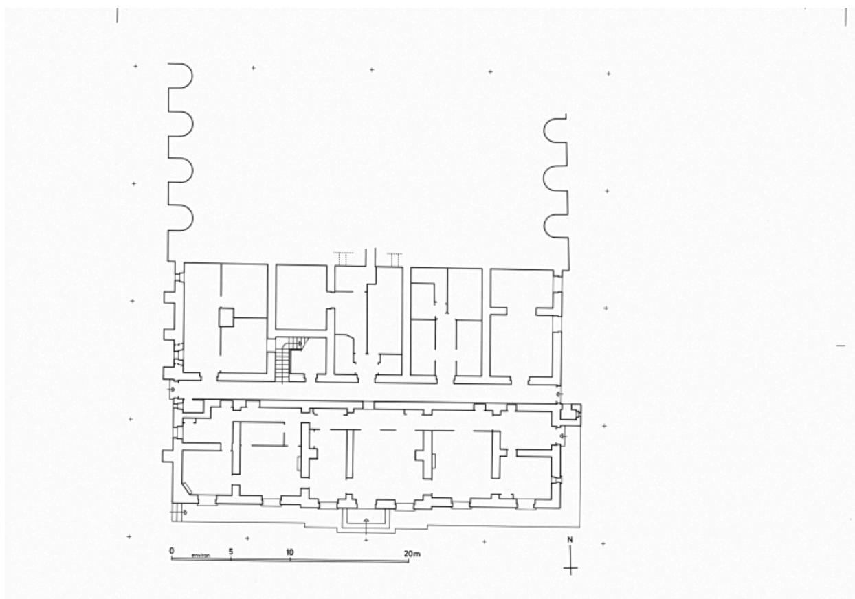
Plan de l'étage de soubassement. Dessin Inventaire P.Chérblanc, 1997, d'après plan anonyme, 1969.
