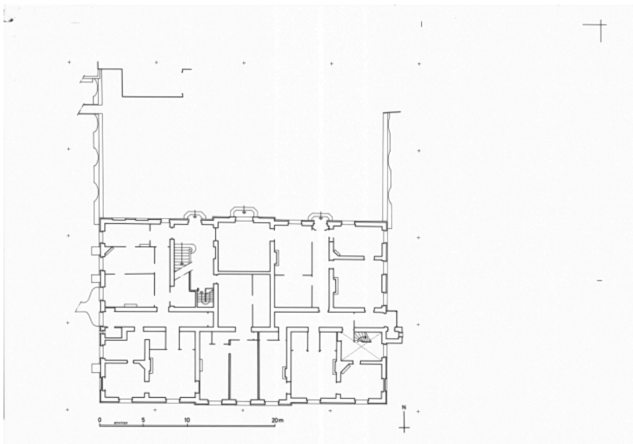
Plan du rez-de-chaussée surélevé. Dessin Inventaire P.Cherblanc, 1997, d'après plan anonyme, 1969.
