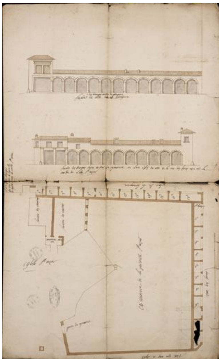
Plan et élévations des boutiques construites en 1564 autour du cimetière, ca 1661
