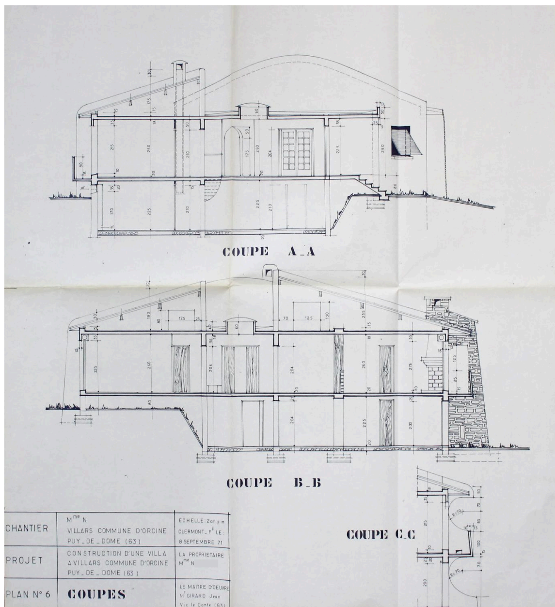
Orcines, la maison N., coupes, Jean Girard maître d'œuvre, septembre 1971 (archives municipales d'Orcines).
