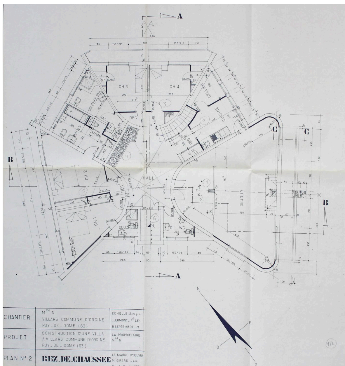
Orcines, la maison N., plan du rez-de-chaussée, Jean Girard maître d'œuvre, septembre 1971 (archives municipales d'Orcines).
