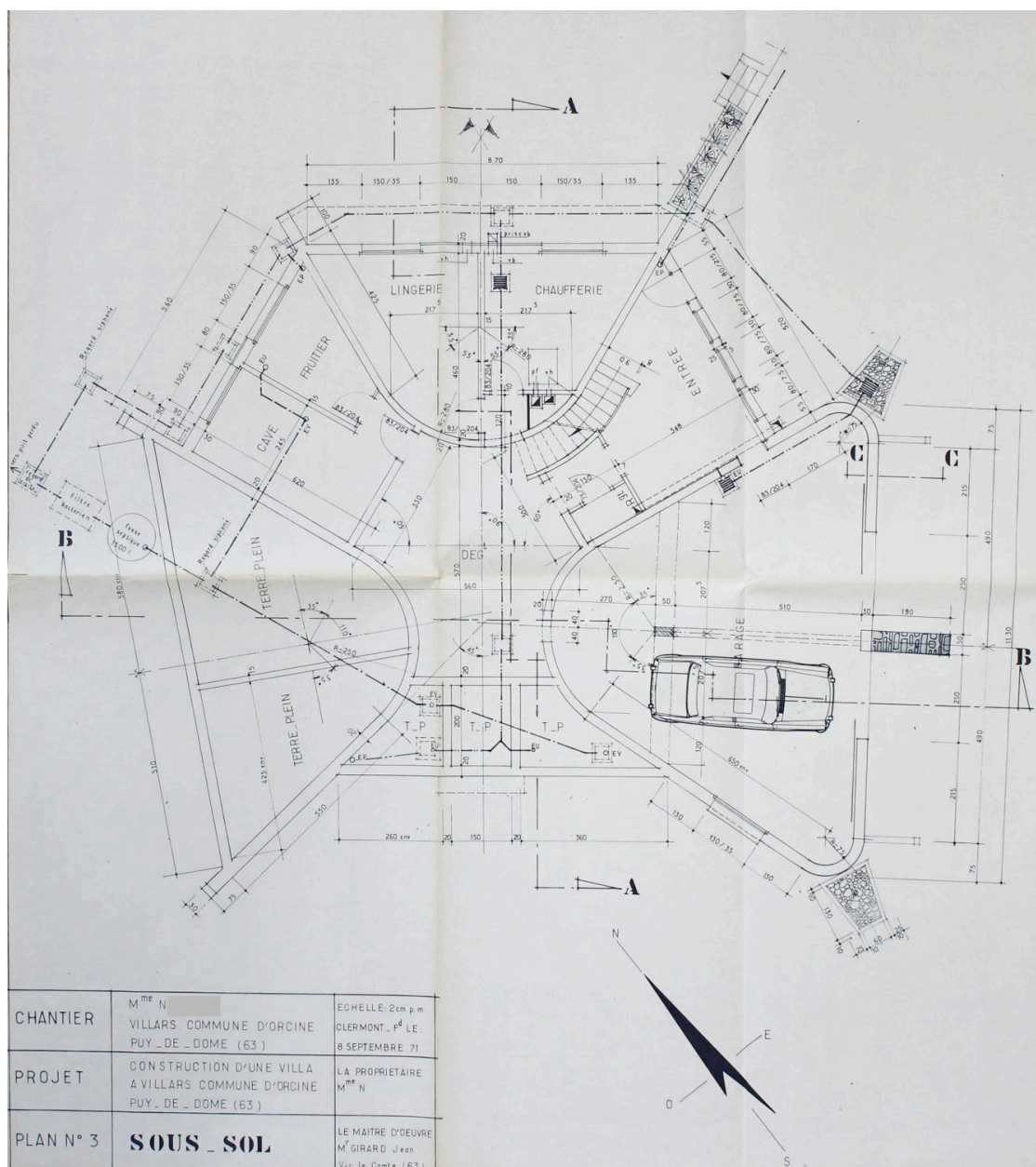
Orcines, la maison N., plan du sous-sol, Jean Girard maître d'œuvre, septembre 1971 (archives municipales d'Orcines).
