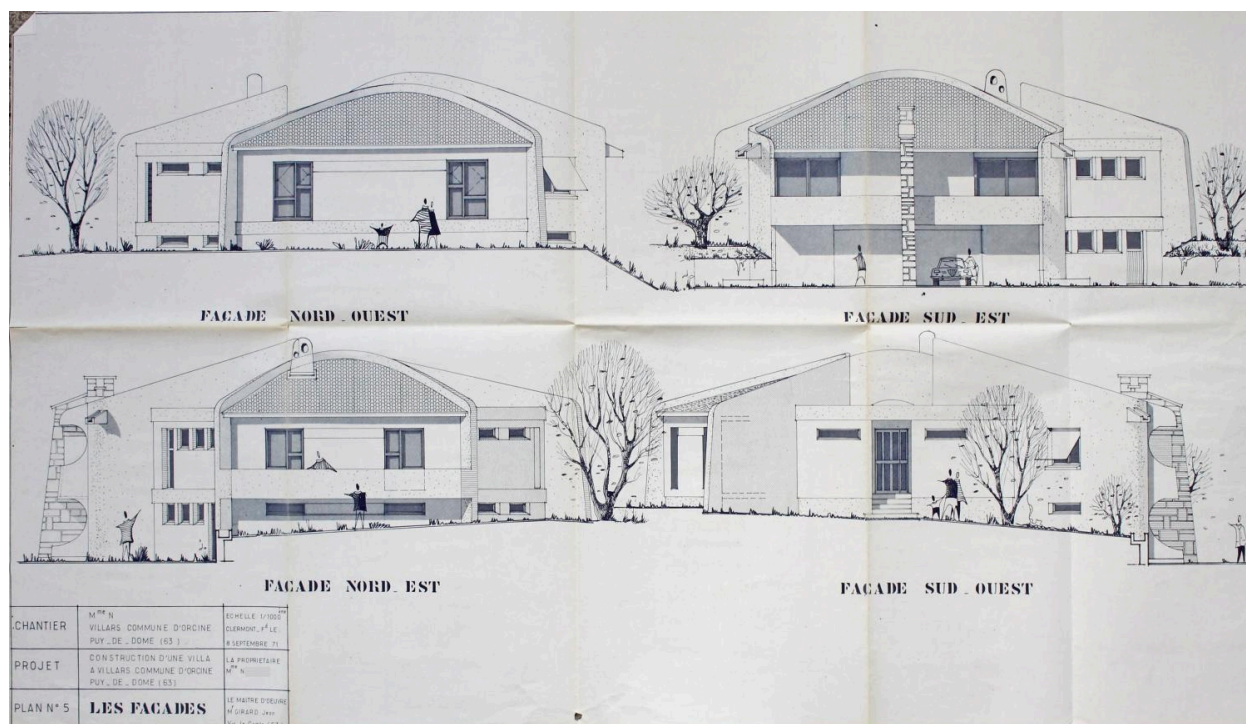
Orcines, la maison N., façades, Jean Girard maître d'œuvre, septembre 1971 (archives municipales d'Orcines).
