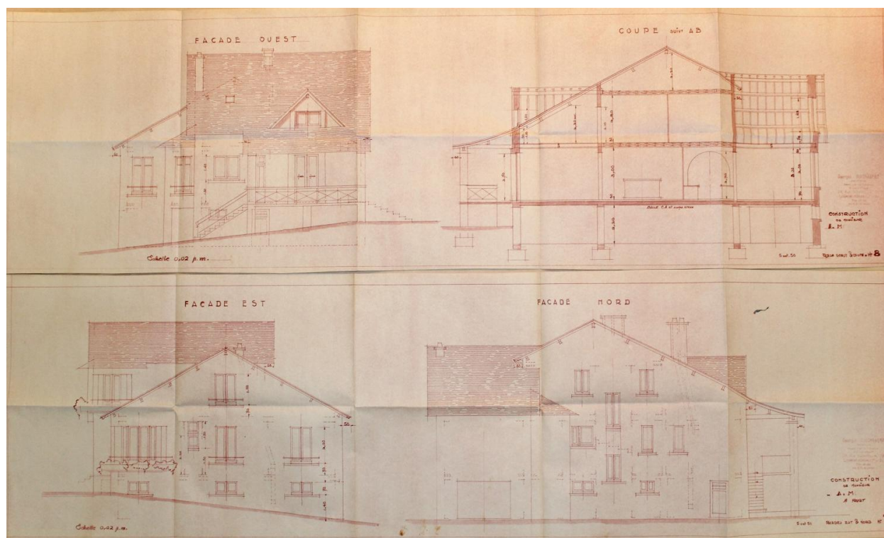
Royat, la maison M., façades ouest, est et nord, coupe A-B, octobre 1950, Georges Guignabert architecte (Archives départementales du Puy-de-Dôme, Fonds de la Direction départementale de l'Équipement, 1611 W 47, PC n° 1822).
