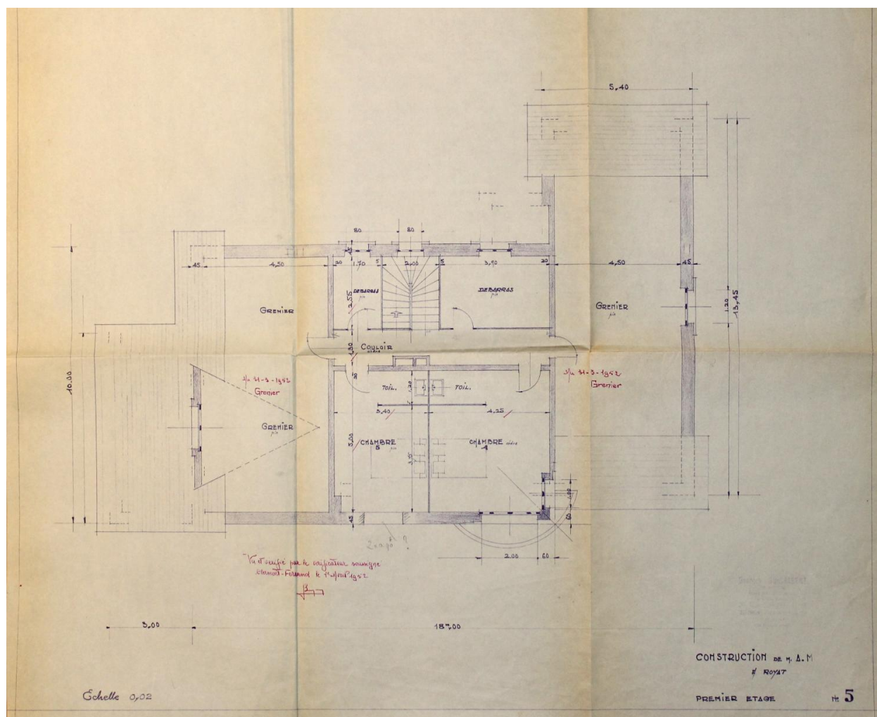
Royat, la maison M., plan de l'étage de comble, octobre 1950, Georges Guignabert architecte (Archives départementales du Puy-de-Dôme, Fonds de la Direction départementale de l'Équipement, 1611 W 47, PC n° 1822).
