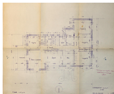
Royat, la maison M., plan du rez-de-chaussée surélevé, octobre 1950, Georges Guignabert architecte (Archives départementales du Puy-de-Dôme, Fonds de la Direction départementale de l'Équipement, 1611 W 47, PC n° 1822). Repro. Christophe Laurent, Autr. Georges Guignabert IVR84_20216302599NUCA
