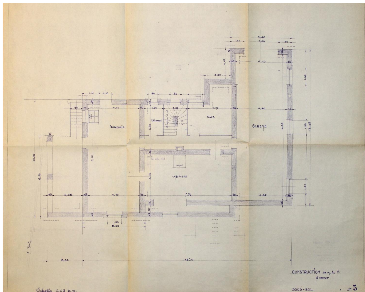
Royat, la maison M., plan du sous-sol semi-enterré, octobre 1950, Georges Guignabert architecte (Archives départementales du Puy-de-Dôme, Fonds de la Direction départementale de l'Équipement, 1611 W 47, PC n° 1822).
