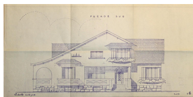
Royat, la maison M., façade principale (sud), octobre 1950, Georges Guignabert architecte (Archives départementales du Puy-de-Dôme, Fonds de la Direction départementale de l'Équipement, 1611 W 47, PC n° 1822). Phot. Christophe Laurent, Autr. Georges Guignabert IVR84_20216302601NUCA
