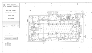
Plan du rez-de-chaussée de l'église Saint-Polycarpe, Marc Charmasson (géomètre), 1999 Autr. Marc Charmasson IVR84_20256900350NUCA
