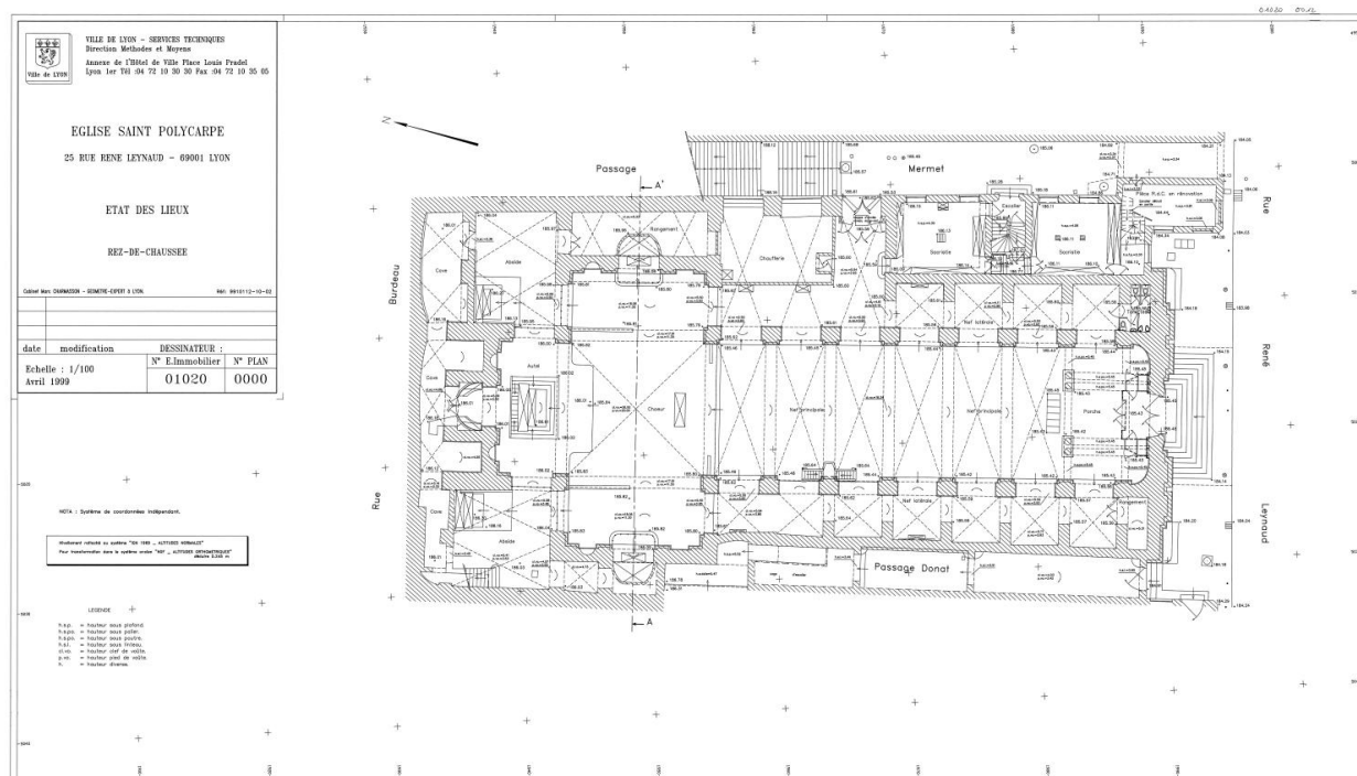
Plan du rez-de-chaussée de l'église Saint-Polycarpe, Marc Charmasson (géomètre), 1999
