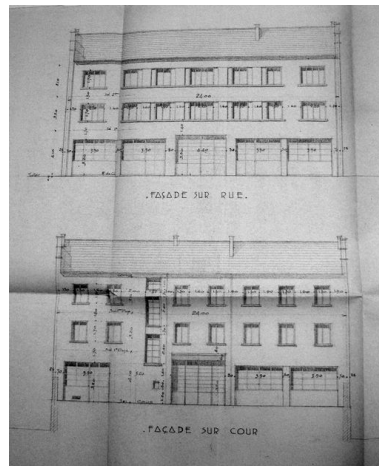
Façades, Immeuble à usage principal d'habitation, 6 rue Challemel Lacour, par Yvon Meunier architecte, échelle 1/100. (Arch. mun. Lyon) Phot. Salohy Rakotomalala IVR82_20106901476NUC
