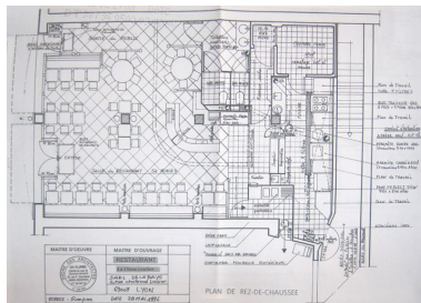
Plan du RDC, Restaurant La Choucrountine, 6 rue Challemel Lacour, 28 mai 1996 par Pluriel architecte échelle 1/20. (Arch. mun. Lyon) Phot. Salohy Rakotomalala IVR82_20106901478NUC
