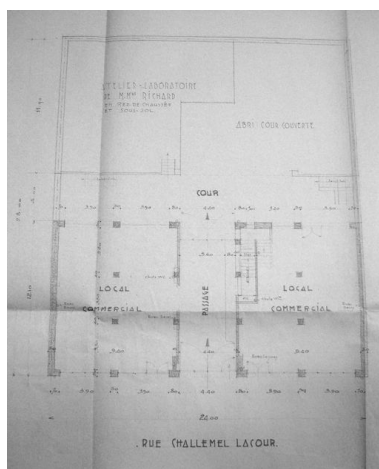
Plan du RDC, Immeuble à usage principal d'habitation, 6 rue Challemel Lacour, par Yvon
