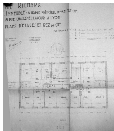
Plans RDC et étages, Immeuble à usage principal d'habitation, 6 rue Challemel Lacour, mai 1954 par Yvon Meunier architecte, échelle 1/100. (Arch. mun. Lyon)
