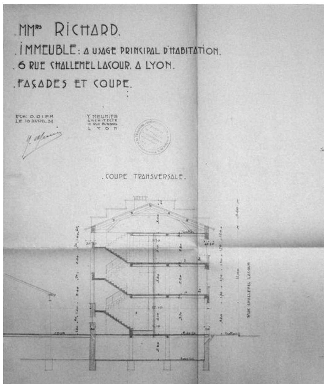
Coupe transversale, Immeuble à usage principal d'habitation, 6 rue Challemeil Lacour, 10 avril 1954 par Yvon Meunier architecte, échelle 1/100. (Arch. mun. Lyon)
