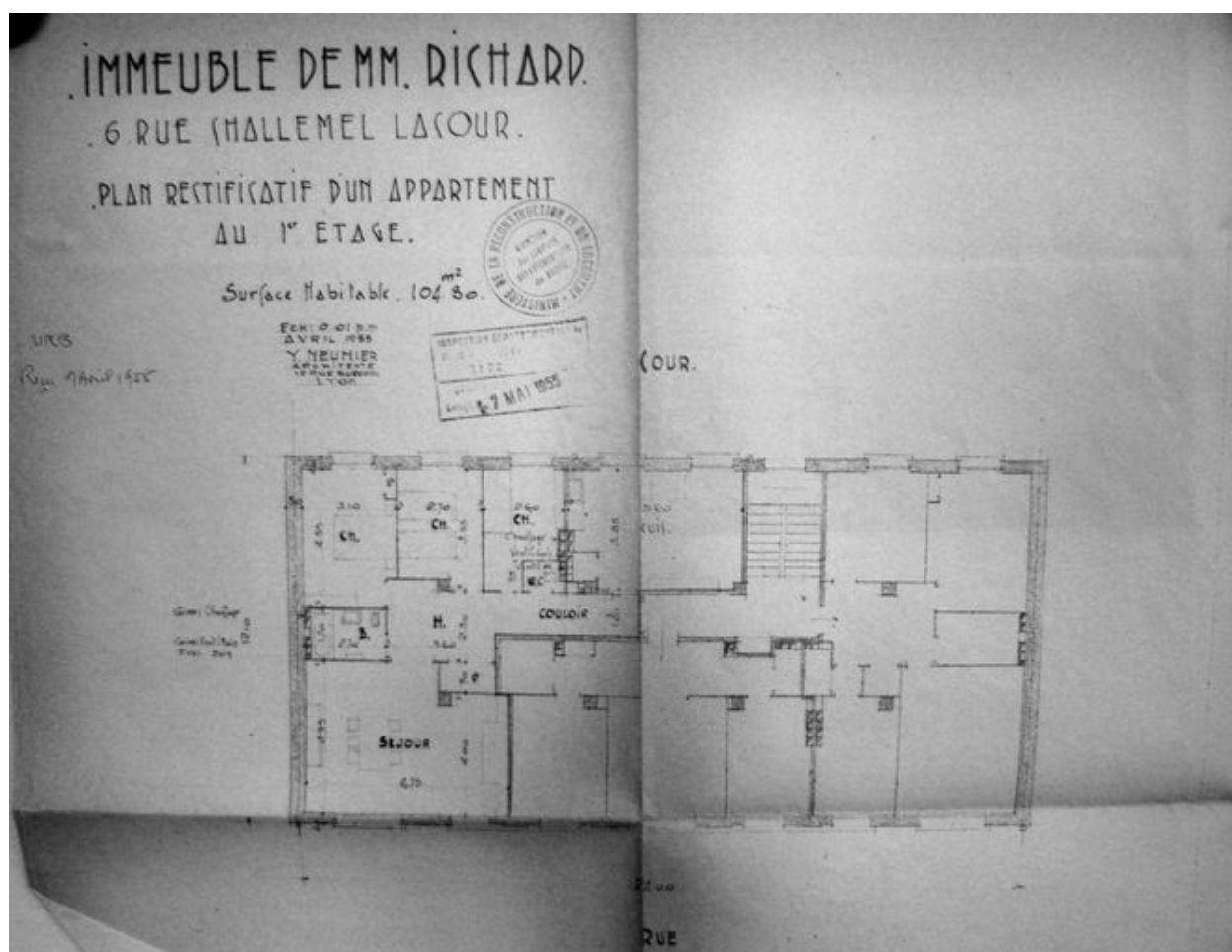
Plan rectificatif d'un appartement au 1er étage, Immeuble à usage principal d'habitation, 6 rue Challemeil Lacour, avril 1955 par Yvon Meunier architecte, échelle 1/100. (Arch. mun. Lyon)
