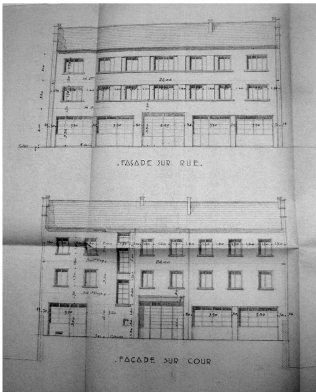
Façades, Immeuble à usage principal d'habitation, 6 rue Challemel Lacour, par Yvon Meunier architecte, échelle 1/100. (Arch. mun. Lyon)
