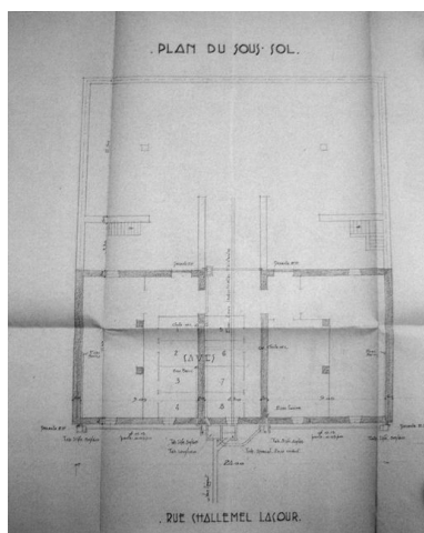
Plan du sous sol, Immeuble à usage principal d'habitation, 6 rue Challemel Lacour, par
