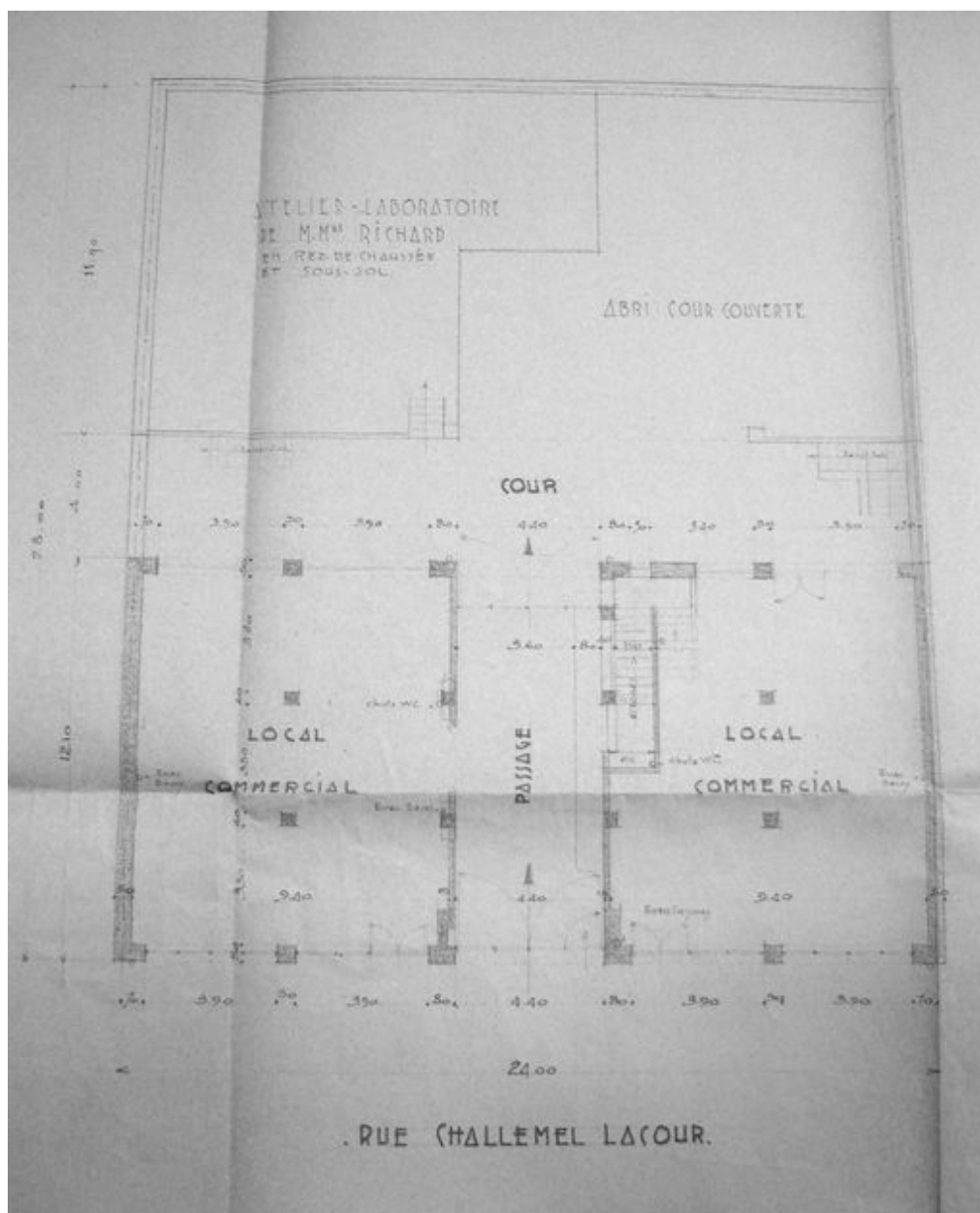
Plan du RDC, Immeuble à usage principal d'habitation, 6 rue Challemeil Lacour, par Yvon Meunier architecte, échelle 1/100. (Arch. mun. Lyon)
