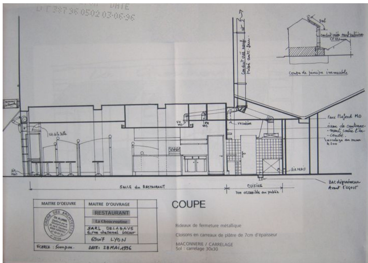
Coupe, Restaurant La Choucroutine, 6 rue Challemel Lacour, 28 mai 1996 par Pluriel architecte, échelle 1/20. (Arch. mun. Lyon)
