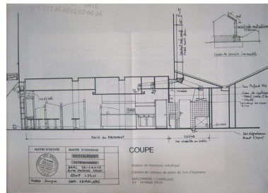
Coupe, Restaurant La Choucrountine, 6 rue Challemel Lacour, 28 mai 1996 par Pluriel architecte, échelle 1/20. (Arch. mun. Lyon) Phot. Salohy Rakotomalala IVR82_20106901479NUC
