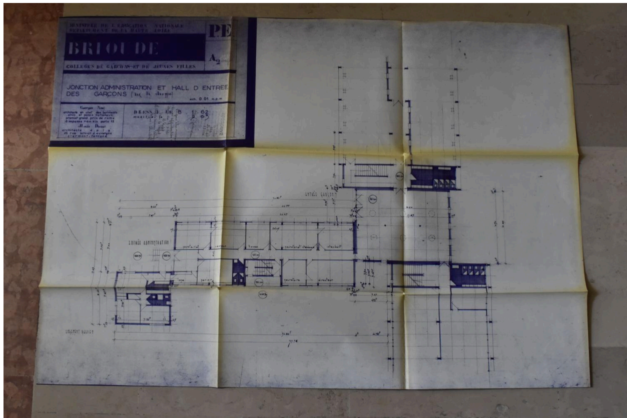
Plan de la jonction entre administration et hall d'entrée des garçons, par G. Noël et J-L. Douat, 8 janvier 1962, modifié en septembre 1963, approuvé en 1966. (AC Brioude. 1 W 1489)
