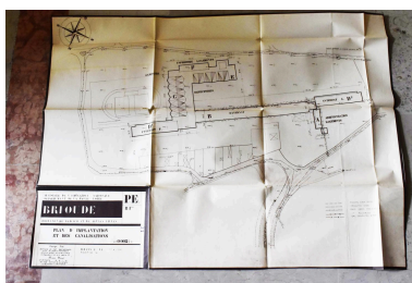
Plan d'implantation et des canalisations, par G. Noël et J-L. Douat, 17 avril 1962 (AC Brioude. 1 W 1489) Repro. Bénédicte Renaud-Morand, Autr. Georges Marie Noël, Autr. Jean-Louis Douat IVR84_20224300081NUCA
