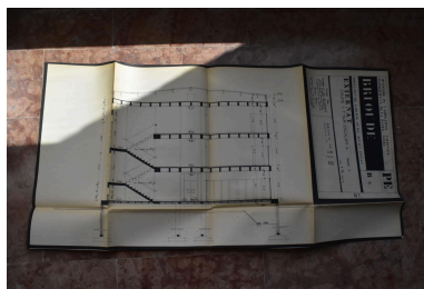
Coupe sur l'escalier nord du bâtiment d'externat, par G. Noël et J.-L. Douat, 8 janvier 1962, modifié le 10 mai 1962 (AC Brioude. 1 W 1489) Repro. Bénédicte Renaud-Morand, Autr. Georges Marie Noël, Autr. Jean-Louis Douat IVR84_20224300082NUCA
