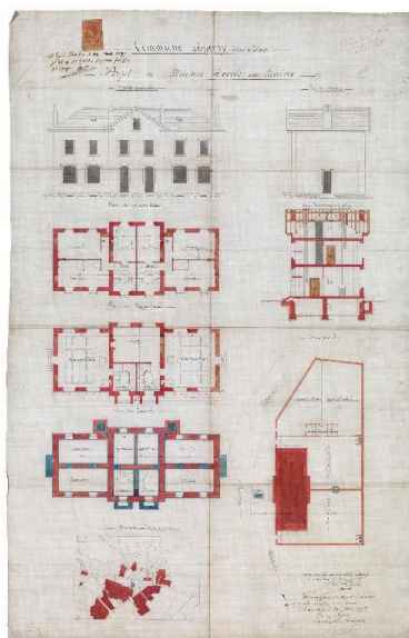
Projet de maison d'école avec mairie, J. de Bons, 1895 (AD Savoie. 2O : 1333). Phot. Thierry Leroy IVR84_20177301788NUCA
