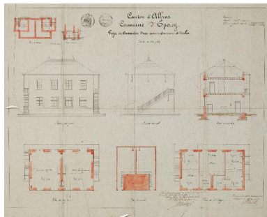
Projet de construction d'une maison commune et d'écoles, J.-S. Revel, 1863 (AD Savoie. 2O : 1332). Phot. Thierry Leroy IVR84_20177301787NUCA
