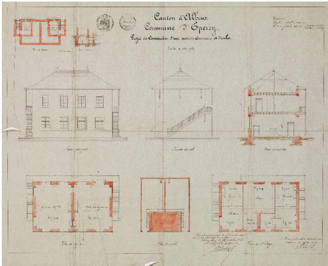
Projet de construction d'une maison commune et d'écoles, J.-S. Revel, 1863 (AD Savoie. 2O : 1332).
