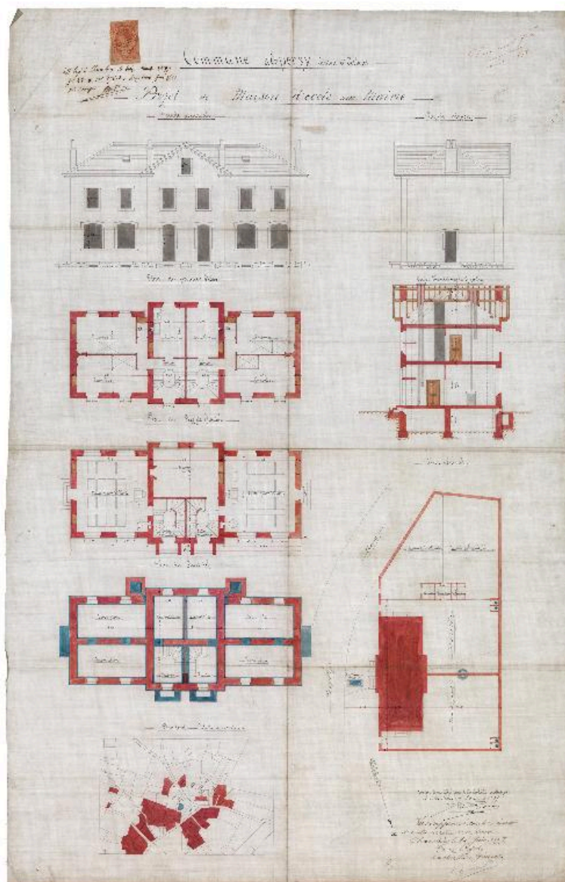
Projet de maison d'école avec mairie, J. de Bons, 1895 (AD Savoie. 2O : 1333).
