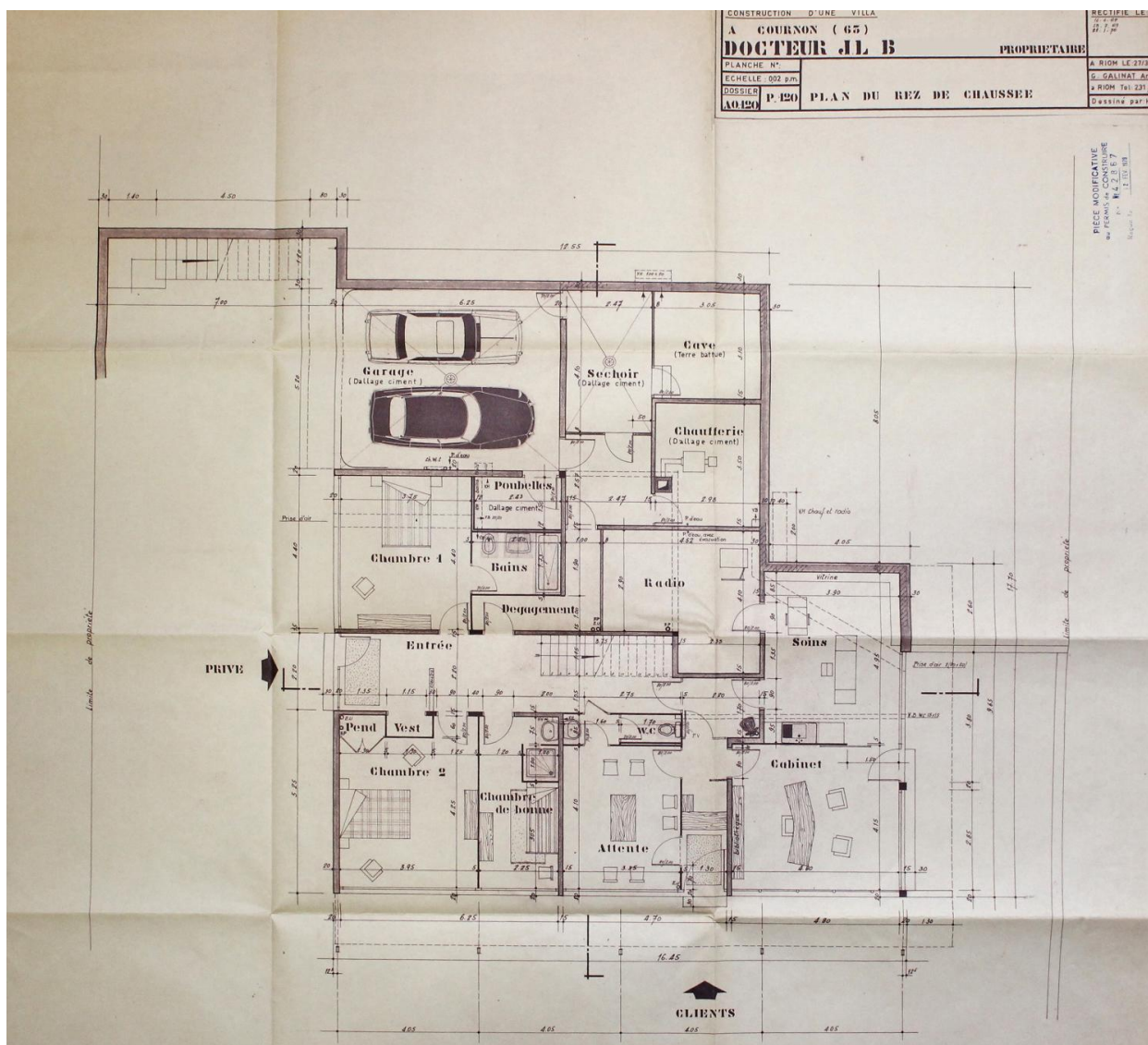
Cournon d'Auvergne, la Maison B., plan du rez-de-chaussée, seconde version, 1969, agence Galinat architectes (archives municipales de Cournon d'Auvergne).
