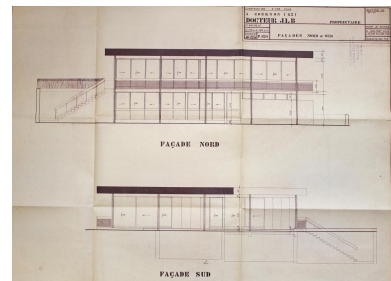
Cournon d'Auvergne, la Maison B., façades nord (principale) et sud, 1969, agence Galinat architectes (archives municipales de Cournon d'Auvergne).
