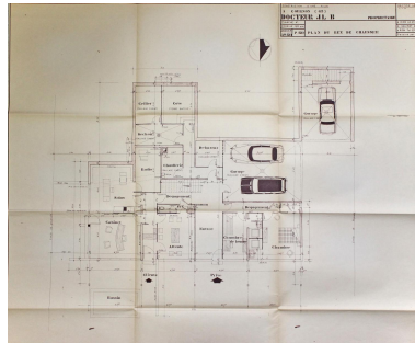
Cournon d'Auvergne, la Maison B., plan du rez-de-chaussée, première version, 1969, agence Galinat architectes (archives municipales de Cournon d'Auvergne).
