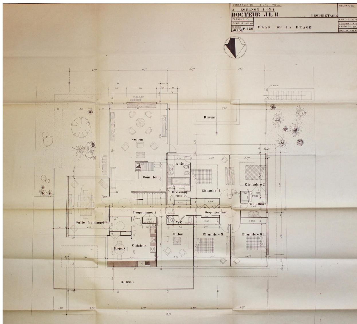
Cournon d'Auvergne, la Maison B., plan du premier étage, première version, 1969, agence Galinat architectes (archives municipales de Cournon d'Auvergne).
