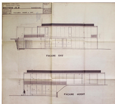
Cournon d'Auvergne, la Maison B., façades est et ouest (latérales), 1969, agence Galinat architectes (archives municipales de Cournon d'Auvergne).
