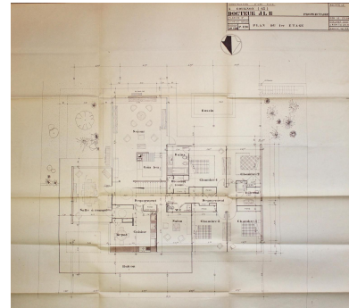
Cournon d'Auvergne, la Maison B., plan du premier étage, première version, 1969, agence Galinat architectes (archives municipales de Cournon d'Auvergne).
