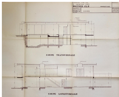
Cournon d'Auvergne, la Maison B., coupes transversale et longitudinale, 1969, agence Galinat architectes (archives municipales de Cournon d'Auvergne).
