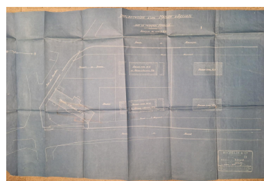
Cité de Blanzat-Beaupeyras : plan masse de la maison d'accueil pour jeunes filles, bleu d'architecte, échelle 0,005 m/m, dessin n° 55.412, s.n., 11/081925. Archives municipales de Clermont-Ferrand, cote 16 A 948.
