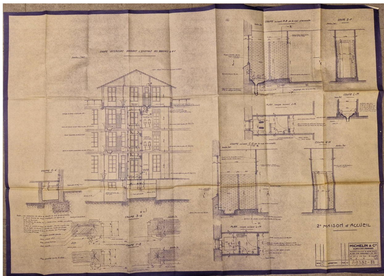
Coupe générale, et coupes de détails sur les sanitaires, du 2e foyer pour jeunes filles, tirage sur papier, échelle 0,02 m/m, dessin n° 69.782, s.n., 25/06/1929. Archives municipales de Clermont-Ferrand, cote 19 A 1346.
