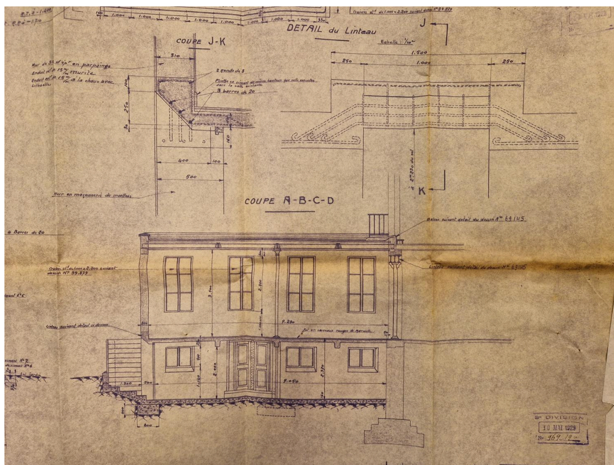
Détail de la coupe du projet d'agrandissement du 1er foyer de jeunes filles, tirage sur papier, dessin n° 69.144, échelle 0,02 m/m, s.n., 15/04/1929. Archives municipales de Clermont-Ferrand, cote 19 A 969.
