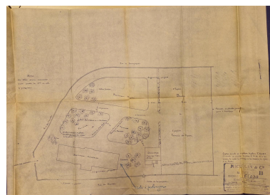
Plan masse avec emplacement du foyer de jeunes filles et indication de la zone où un agrandissement est à prévoir, tirage sur papier, échelle 0,005 m/m, s.n., s.d. [1929 ? / 1927 pour le fond de plan]. Archives municipales de Clermont-Ferrand, cote 19 A 969. Repro. Brigitte Ceroni IVR84_20236300753NUCA
