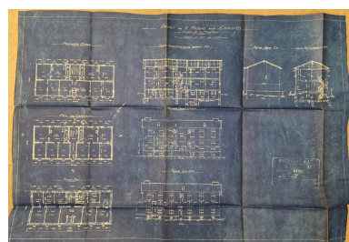
Plans, coupes et élévations du projet de la cité de Blanzat- Beaupeyras, bleu d'architecte, échelle 0,010 m/m, dessin n° 49.271, s.n., 12/10/1923. Archives municipales de Clermont-Ferrand, cote 16 A 948.
