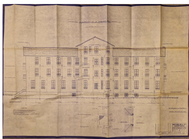
Élévation est cotée du 2e foyer pour jeunes filles, tirage sur papier, échelle 0,02 m/m, dessin n° 69.912, s.n., 08/07/1929. Archives municipales de Clermont-Ferrand, cote 19 A 1346. Repro. Brigitte Ceroni IVR84_20236300750NUCA
