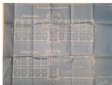
Plans des 3e et 4e étages du foyer pour jeunes filles, bleu d'architecte, échelle 0,02 m/ m, dessin n° 55.411, s.n., 18/08/1925. Archives municipales de Clermont-Ferrand, cote 17 A 950.
