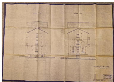
Élévations nord et sud cotées du 2e foyer pour jeunes filles, tirage sur papier, échelle 0,02 m/m, dessin n° 69.914, s.n., 08/07/1929. Archives municipales de Clermont-Ferrand, cote 19 A 1346. Repro. Brigitte Ceroni IVR84_20236300751NUCA
