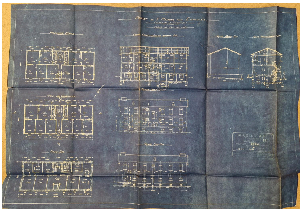
Plans, coupes et élévations du projet de la cité de Blanzat-Beaupeyras, bleu d'architecte, échelle 0,010 m/m, dessin n° 49.271, s.n., 12/10/1923. Archives municipales de Clermont-Ferrand, cote 16 A 948.
