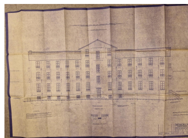
Élévation ouest cotée du 2e foyer pour jeunes filles, tirage sur papier, échelle 0,02 m/m, dessin n° 69.913, s.n., 08/07/1929. Archives municipales de Clermont-Ferrand, cote 19 A 1346. Repro. Brigitte Ceroni IVR84_20236300773NUCA
