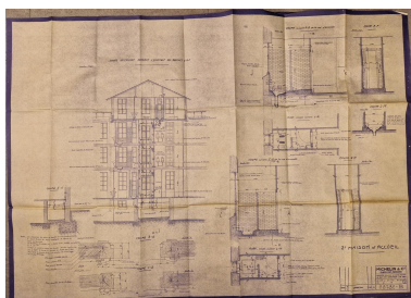
Coupe générale, et coupes de détails sur les sanitaires, du 2e foyer pour jeunes filles, tirage sur papier, échelle 0,02 m/m, dessin n° 69.782, s.n., 25/06/1929. Archives municipales de Clermont-Ferrand, cote 19 A 1346. Repro. Brigitte Ceroni IVR84_20236300752NUCA
