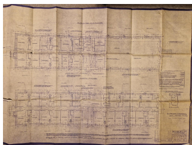
Plans cotés du rez-de-chaussée et du 1er étage du 2e foyer pour jeunes filles, tirage sur papier, échelle 0,02 m/m, dessin n° 69.154, s.n., 16/04/1929. Archives municipales de Clermont-Ferrand, cote 19 A 1346. Repro. Brigitte Ceroni IVR84_20236300749NUCA
