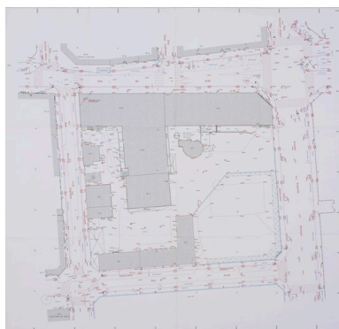
Plan topographique, SERL, échelle 1/200 Phot. Eric Dessert IVR82_20056902985NUCA
