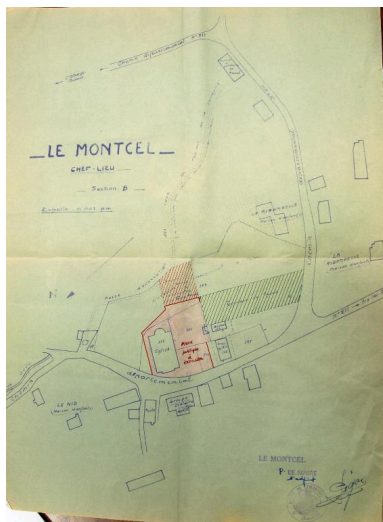
Commune de LE MONTCEL. Construction d'une place publique. Plan général au 1/1000e. M. Michel, ingénieur T.P.E., 6 mai 1950.
