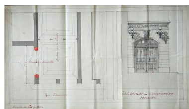
Projet de porte pour le théâtre Bouffes-Scala, 1899
