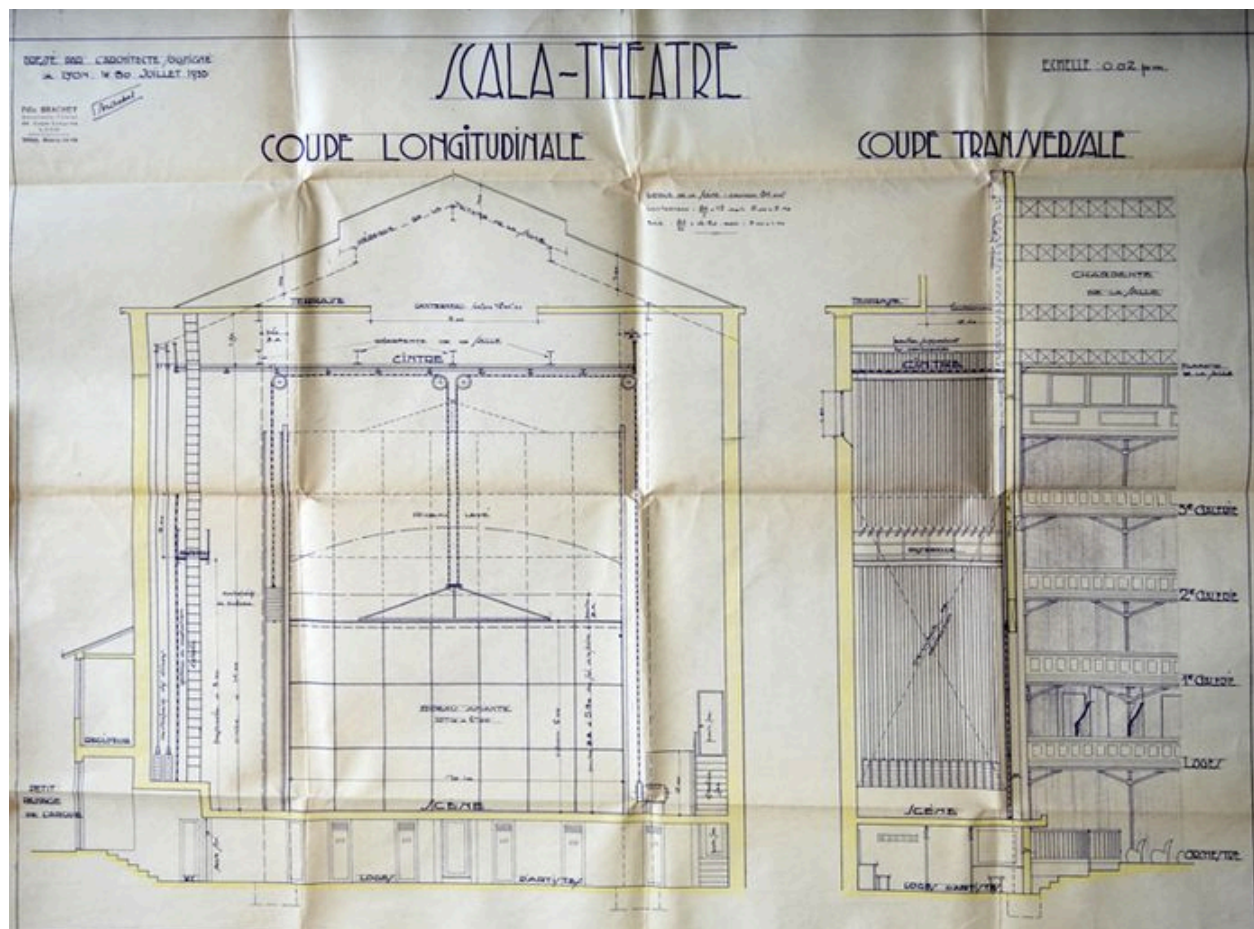
Projet de transformation de l'architecte Félix Brachet, 1933 : coupes longitudinale et transversale
