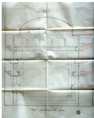
Coupe par le devant de la scène, 1880 ca.
