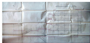
Coupe longitudinale, 1880 ca.
