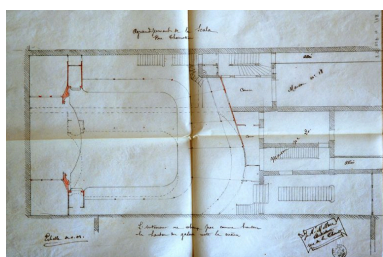
Projet d'agrandissement, 1884 ca.
