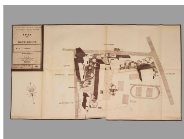
Plan masse, 30 janvier 1960, modifié le 24/3/1960, modifié le 2/4/1960. Phot. Christian Parisey IVR84_20206300522NUC4A
