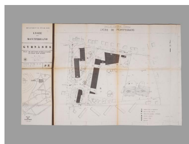
Plan de situation des gymnases, 13/3/1967, modifié le 22/9/1967. La tour d'escalier hors-oeuvre implantée au nord-ouest de la parcelle est indiquée (mais son plan n'est pas exact) contrairement au plan d'exécution daté de 1961 qui ne la représentait pas du tout. Phot. Christian Parisey IVR84_20206300526NUC4A
