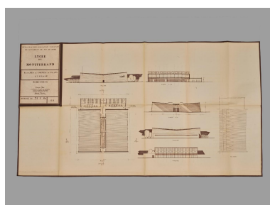
Façades-coupes-plans du gymnase, 31/1/1960. Projet non réalisé.
