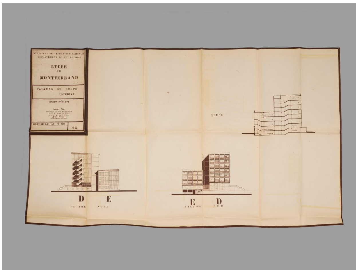
Façades et coupe. Internat. AU 31/1/1960.
