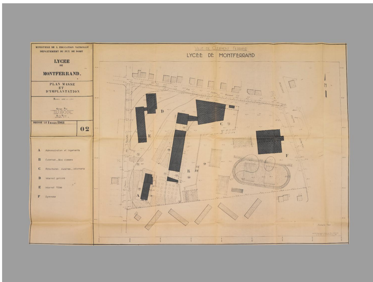
Plan masse et d'implantation, 1er/3/1961.
