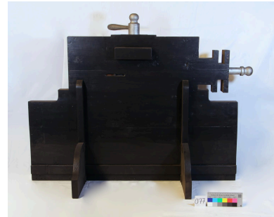
Modèle de distribution de vapeur, vue arrière Phot. Krystelle Besson , Phot. Mirco Meier, Phot. Marion Petit IVR84_20256901122NUCA
