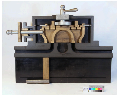
Modèle de distribution de vapeur, vue de face Phot. Krystelle Besson , Phot. Mirco Meier, Phot. Marion Petit IVR84_20256901121NUCA
