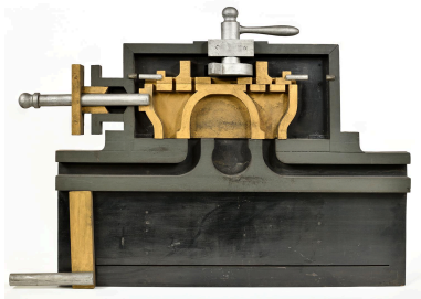
Maquette de distribution de vapeur Phot. Thierry Leroy IVR84_20256901859NUCA
