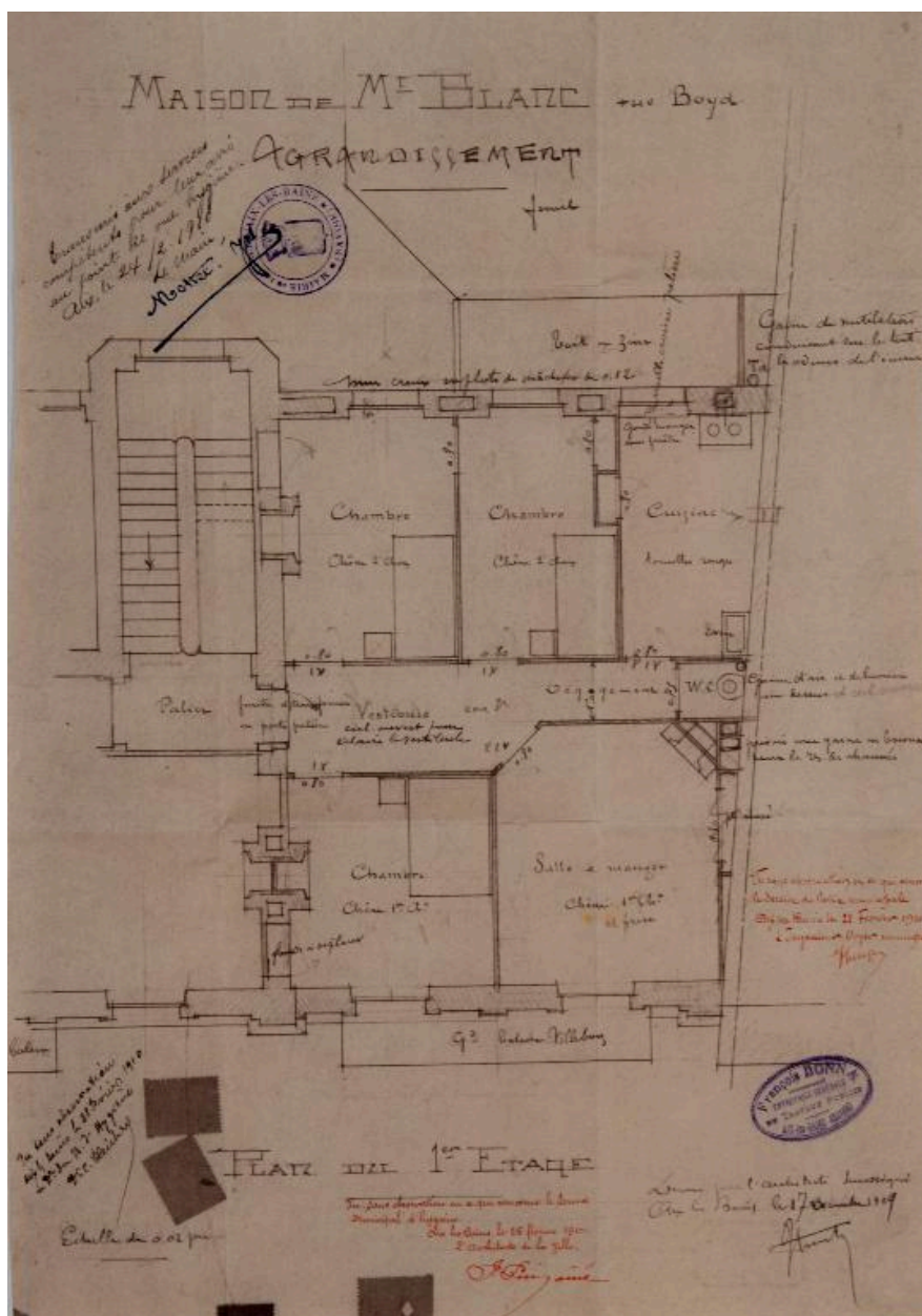
Agrandissement, 1909 : plan du 1er étage
