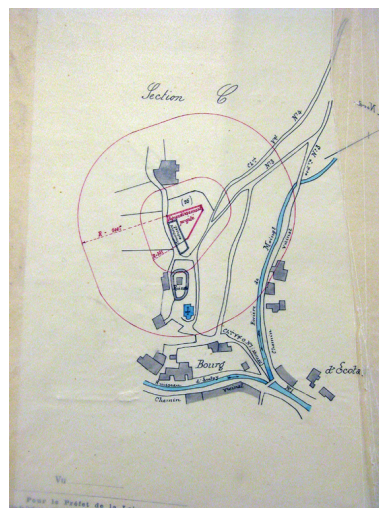
Projet d'agrandissement du cimetière. Plan détaillé des lieux (n°1). Plan sur calque, 1904. AD Loire. O 972. Phot. Thierry Monnet, Autr. Joseph Jaccon IVR82_20124201859NUCA
