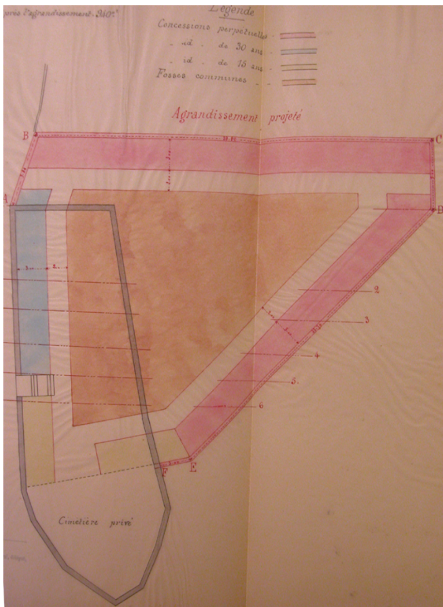
Projet d'agrandissement du cimetière. Plan et profils des travaux projetés (n°2). Plan sur calque, 1904. AD Loire. O 972
