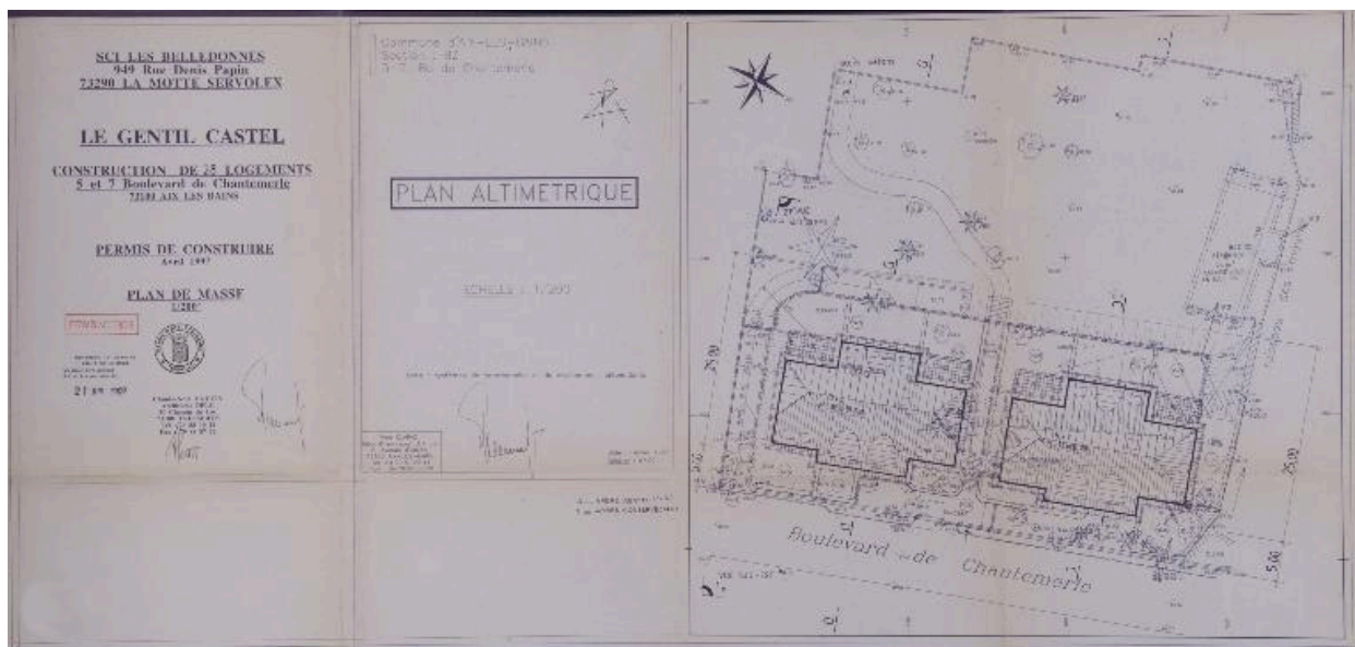
Plan de masse, bac de rétention des nouveaux immeubles, 1997
