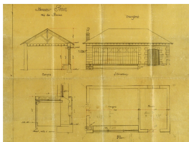
Plan, coupe et élévation Repro. François Fouger IVR82_20077300177NUCB
