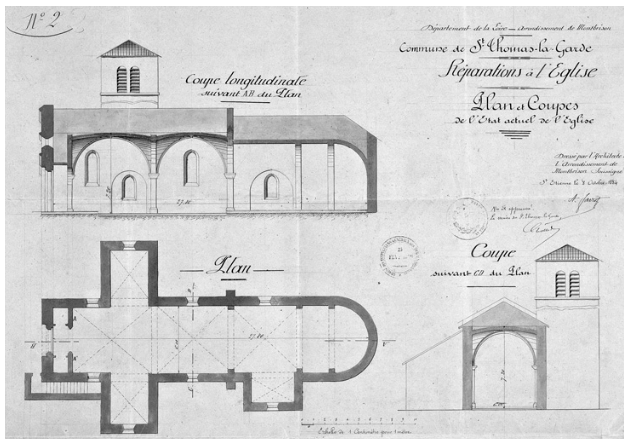
N°2. Réparations à l'église. Plans et coupes de l'état actuel de l'église [1884].
