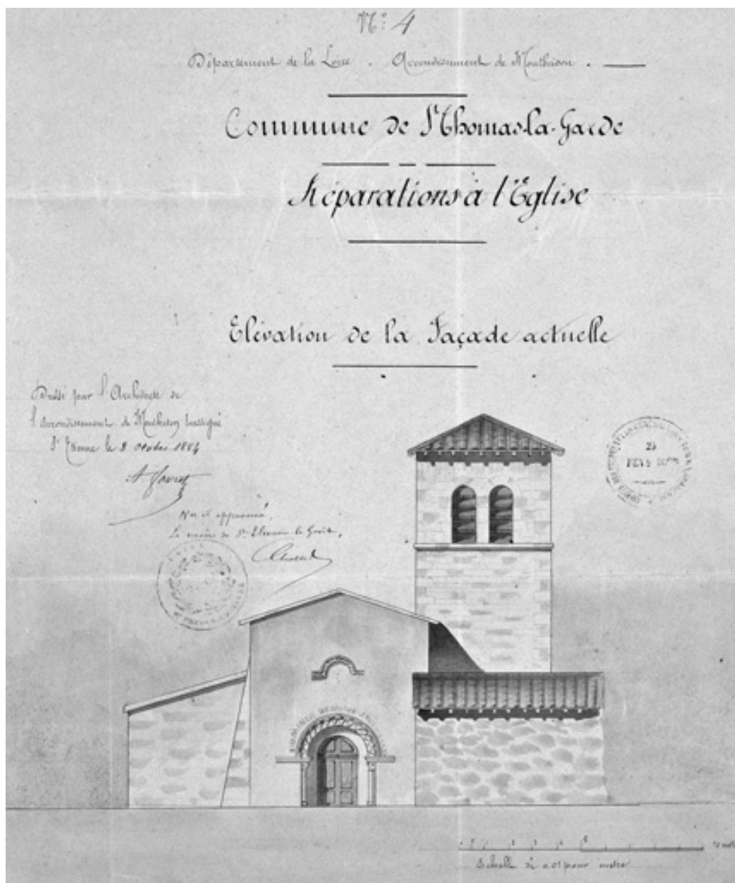
N°4. Réparations à l'église. Elévation de la façade actuelle [1884].
