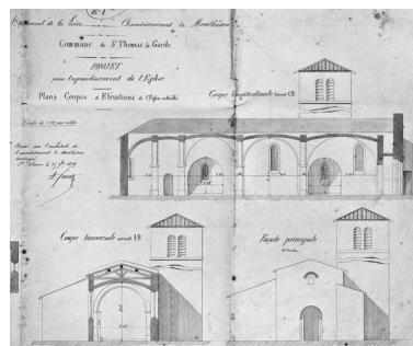
N°1. Projet pour l'agrandissement de l'église. Plans. Coupes et élévations de l'église actuelle. Coupe transversale suivant AB. Coupe longitudinale suivant CD. Façade principale actuelle [1879]. Phot. Eric Dessert, Autr. A. Favrot IVR82_20064200742NUC
