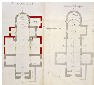
N°1. Projet pour l'agrandissement de l'église. Plans. Coupes et élévations de l'église actuelle. Plan de l'église agrandie. Plan actuel de l'église [1879]. Phot. Eric Dessert, Autr. A. Favrot IVR82_20064200743NUCA
