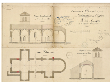
N°3. Restauration de l'église. Plans et coupes de l'église réparée [1884]. Phot. Eric Dessert, Autr. A. Favrot IVR82_20064200746NUC
