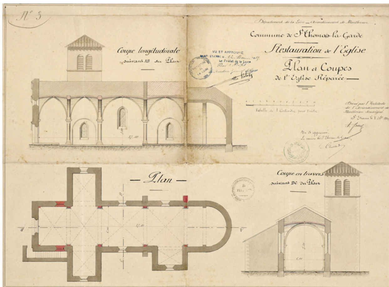
N°3. Restauration de l'église. Plans et coupes de l'église réparée [1884].
