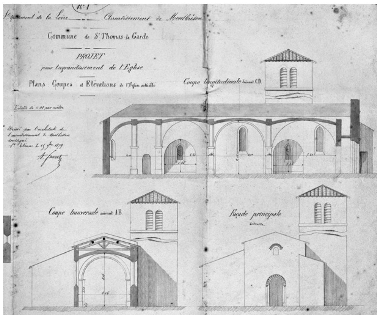
N°1. Projet pour l'agrandissement de l'église. Plans. Coupes et élévations de l'église actuelle. Coupe transversale suivant AB. Coupe longitudinale suivant CD. Façade principale actuelle [1879].
