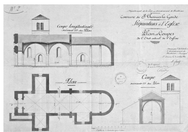
N°2. Réparations à l'église. Plans et coupes de l'état actuel de l'église [1884]. Phot. Eric Dessert, Autr. A. Favrot IVR82_20064200744NUC
