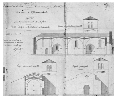
N°1. Projet pour l'agrandissement de l'église. Plans. Coupes et élévations de l'église actuelle. Coupe transversale suivant AB. Coupe longitudinale suivant CD. Façade principale actuelle [1879]. Phot. Eric Dessert, Autr. A. Favrot IVR82_20064200742NUC
