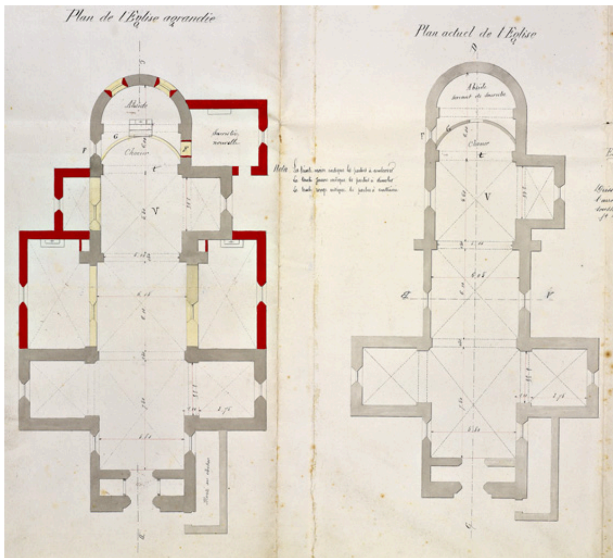
N°1. Projet pour l'agrandissement de l'église. Plans. Coupes et élévations de l'église actuelle. Plan de l'église agrandie. Plan actuel de l'église [1879].
