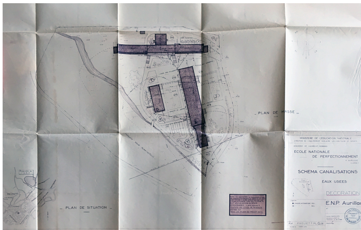
Plan masse avec implantation de la décoration par Louis Cazelles, architecte (AN, 19880466/82)
