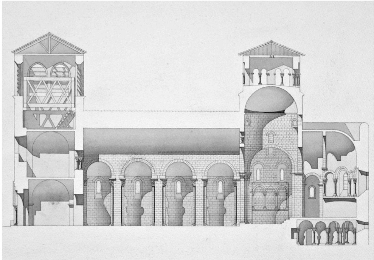
[Coupe longitudinale].
