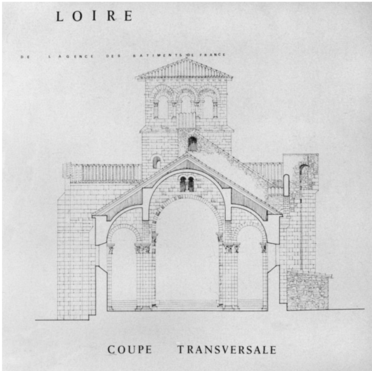
Coupe transversale.
