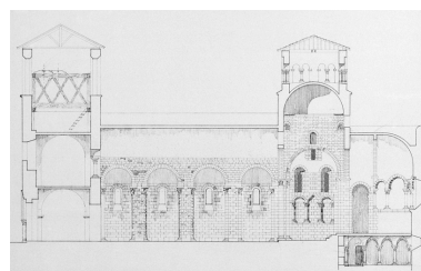
Coupe longitudinale. Phot. Eric Dessert IVR82_20064200765NUC
