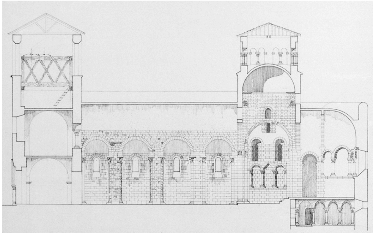
Coupe longitudinale.
