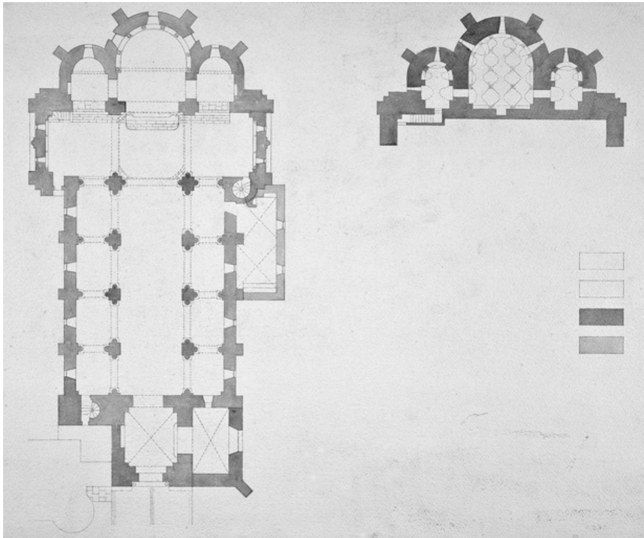
[Plan chronologique de l'édifice ; plan de la crypte].
