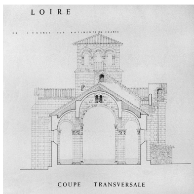
Coupe transversale. Phot. Eric Dessert IVR82_20064200764NUC
