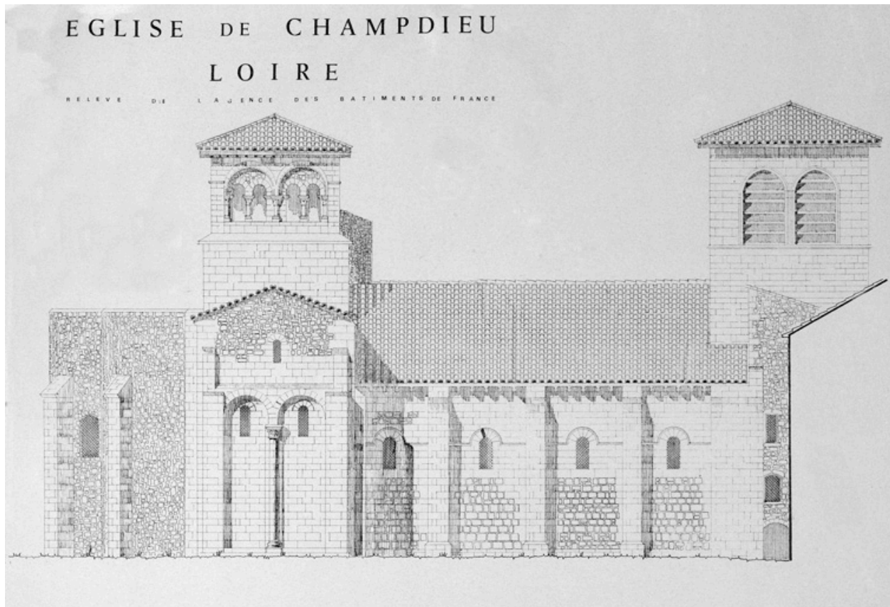
[Relevé de la façade nord.]
