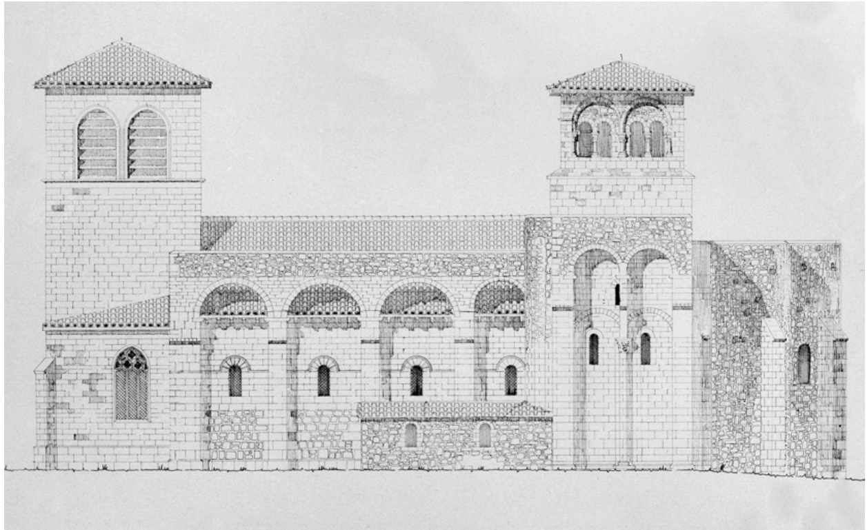
[Relevé de la façade sud.]
