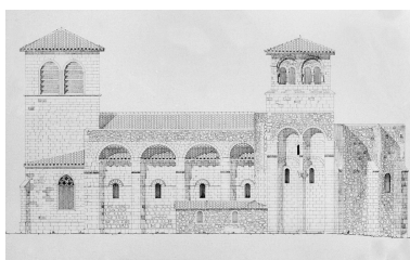
[Relevé de la façade sud.] Phot. Eric Dessert IVR82_20064200768NUC
