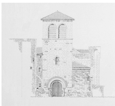
[Relevé de la façade ouest]. Phot. Eric Dessert IVR82_20064200769NUC
