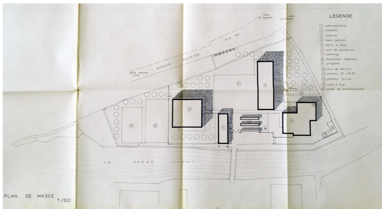
Plan de masse par R. Poirier, 1967 (AN, 19930607/6)
