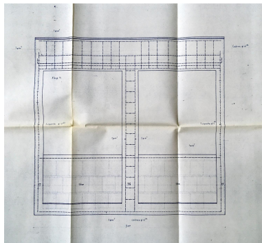
Procédé FIORIO : panneau de façade type avec fenêtre (AN, 19930607/6) Autr. René Poirier, Repro. Catherine Guégan IVR84_20220700201NUCA
