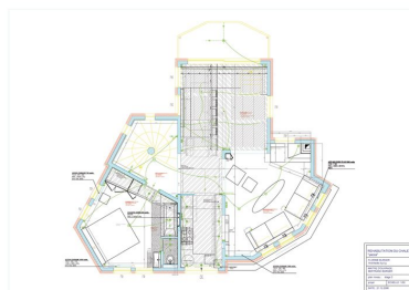
Réhabilitation du chalet Yacca. Plan niveau étage 2. Projet / Florine Burger, 21 décembre 2006 Phot. Jean-François Lyon-Caen, Phot. C. Salomon-Pelen, Autr. Burger Florine (architecte) IVR82_20087400024NUCA
