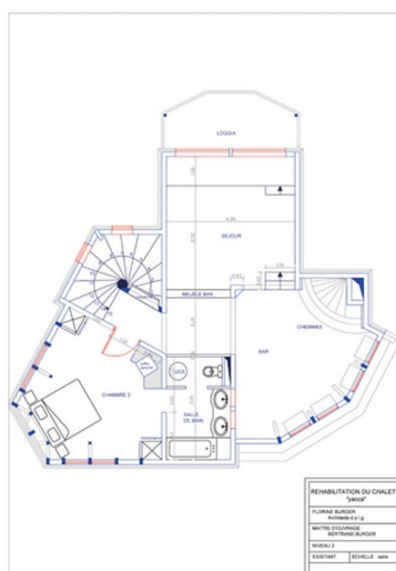
Réhabilitation du chalet Yacca. Plan du niveau 2. Etat avant transformation [séjour] / Florine Burger, 2007 Phot. Jean-François Lyon-Caen, Phot. C. Salomon-Pelen, Autr. Burger Florine (architecte) IVR82_20087400021NUCA
