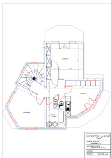
Réhabilitation du chalet Yacca. Plan du niveau 1. Etat avant transformation [chambres] / Florine Burger, 2007 Phot. Jean-François Lyon-Caen, Phot. C. Salomon-Pelen, Autr. Burger Florine (architecte) IVR82_20087400020NUCA
