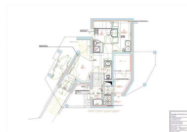
Réhabilitation du chalet Yacca. Plan du niveau RDC. Projet / Florine Burger, 10 août 2007 Phot. Jean-François Lyon-Caen, Phot. C. Salomon-Pelen, Autr. Burger Florine (architecte) IVR82_20087400022NUCA
