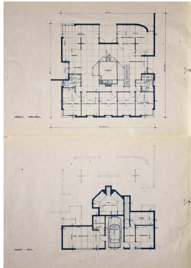
Romagnat, la Maison R., plans du sous-sol partiel semi-enterré et du second niveau, 1973, Michel Mangematin architecte, Jean Porte collaborateur (Archives municipales de Romagnat). Repro. Christophe Laurent, Autr. Michel Mangematin IVR84_20216302471NUCA
