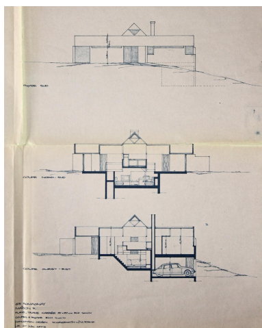
Romagnat, la Maison R., façade sud, coupes nord-sud et est- ouest, 1973, Michel Mangematin architecte, Jean Porte collaborateur (Archives municipales de Romagnat).
