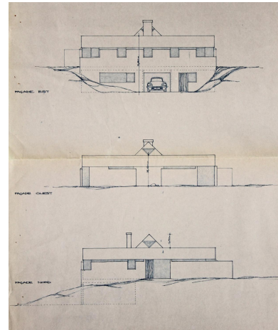
Romagnat, la Maison R., la façade est (principale) et les façades nord et ouest, 1973, Michel Mangematin architecte, Jean Porte collaborateur (Archives municipales de Romagnat). Repro. Christophe Laurent, Autr. Michel Mangematin IVR84_20216302472NUCA
