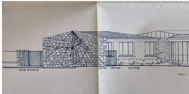
Projet d'exécution par B. Danis, 1961 : détail du mur pignon du pavillon du concierge (AN, 19880466/48) Repro. Catherine Guégan, Autr. Benoît Danis IVR84_20240300448NUCA
