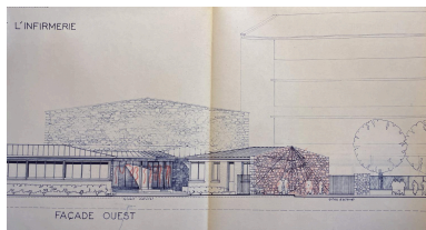
Projet d'exécution pour le collège par B. Danis, 1961 : façade ouest avec esquisse des décorations (en rouge) (AN, 19880466/48) Repro. Catherine Guégan IVR84_20240300207NUCA
