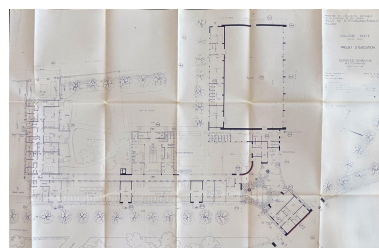
Projet d'exécution : plan du rez-de-chaussée des services généraux avec localisation des décorations (en rouge) (AN, 19880466/48) Repro. Catherine Guégan, Autr. Benoît Danis IVR84_20240300446NUCA
