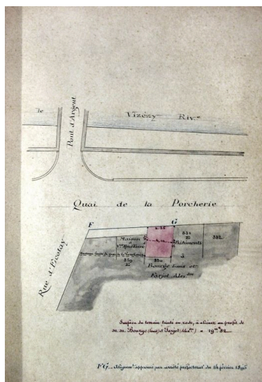
Plan d'alignement sur le quai de la Porcherie, 1895 (AD 42 : série O 1069). plan d'alignement, 1895 AD Loire. O 1069 Phot. Simone Hartmann-Nussbaum IVR82_20114201348NUCA
