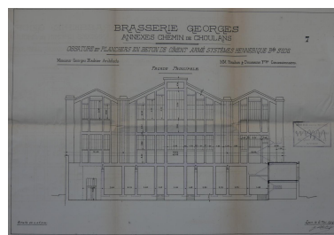
Façade Annexes Choulans Brasseries Georges 1919 (ACL 314W616-207) Phot. Nadine Halitim-Dubois IVR84_20266900350NUCA
