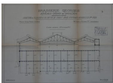
Ossature et planchers Annexes Choulans Brasseries Georges 1919 (ACL 314W616-207) Phot. Nadine Halitim-Dubois IVR84_20266900352NUCA
