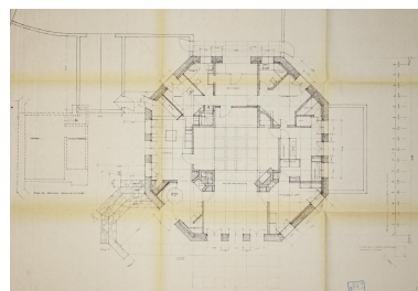
Pont-du-Château, la maison F., plan du sous-sol et du rez-de-chaussée, Michel Mangematin architecte, juillet 1975 (Archives municipales de Pont-du-Château). Repro. Christophe Laurent, Autr. Michel Mangematin IVR84_20216302540NUCA
