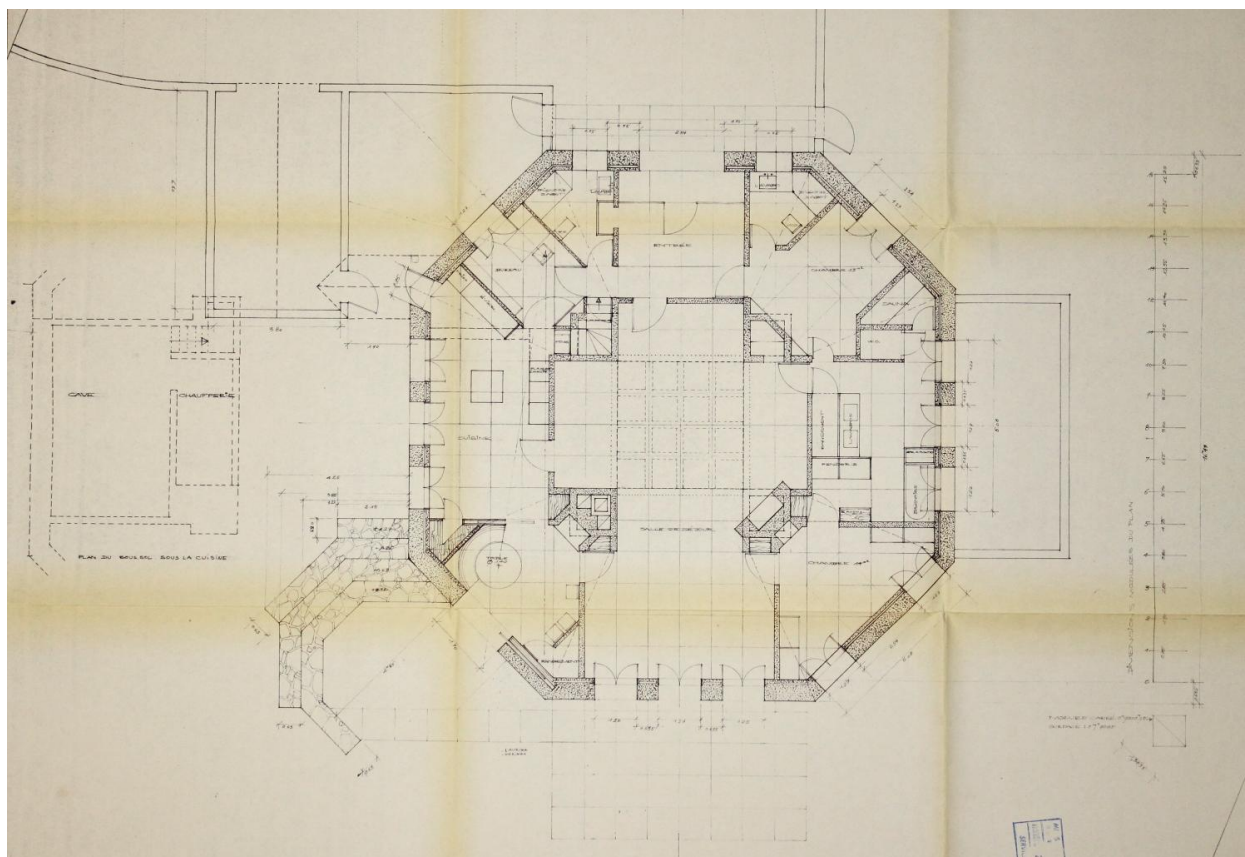
Pont-du-Château, la maison F., plan du sous-sol et du rez-de-chaussée, Michel Mangematin architecte, juillet 1975 (Archives municipales de Pont-du-Château).
