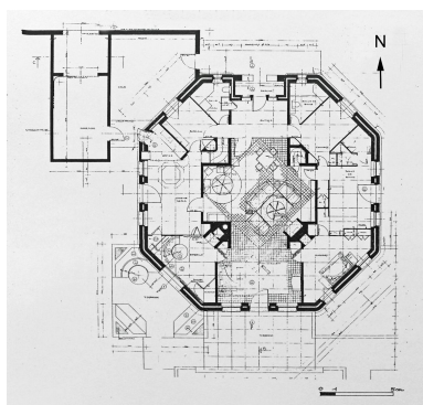
Pont-du-Château, la maison F.*, plan du rez-de-chaussée publié dans Michel Mangematin et alli, Lieux d'être (Paris, Archibooks - Sautereau éditeur, 2011, 152 p.), page 88. Repro. Christophe Laurent, Autr. Michel Mangematin IVR84_20216302541NUCA
