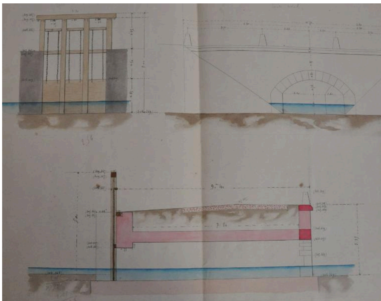
Plan de la prise d'eau, 1866 (FR.AD073, 49SPC2).
