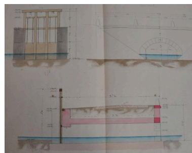
Plan de la prise d'eau, 1866 (FR.AD073, 49SPC2). Autr. Clara Bérelle IVR82_20157301733NUCA
