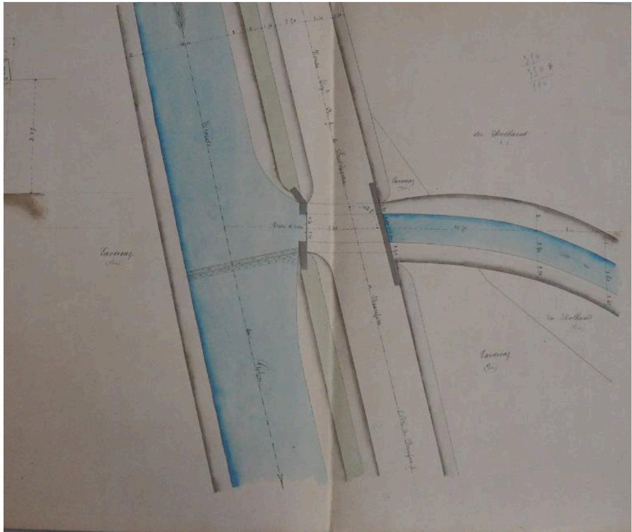
Plan de la prise d'eau, 1866 (FR.AD073, 49SPC2).
