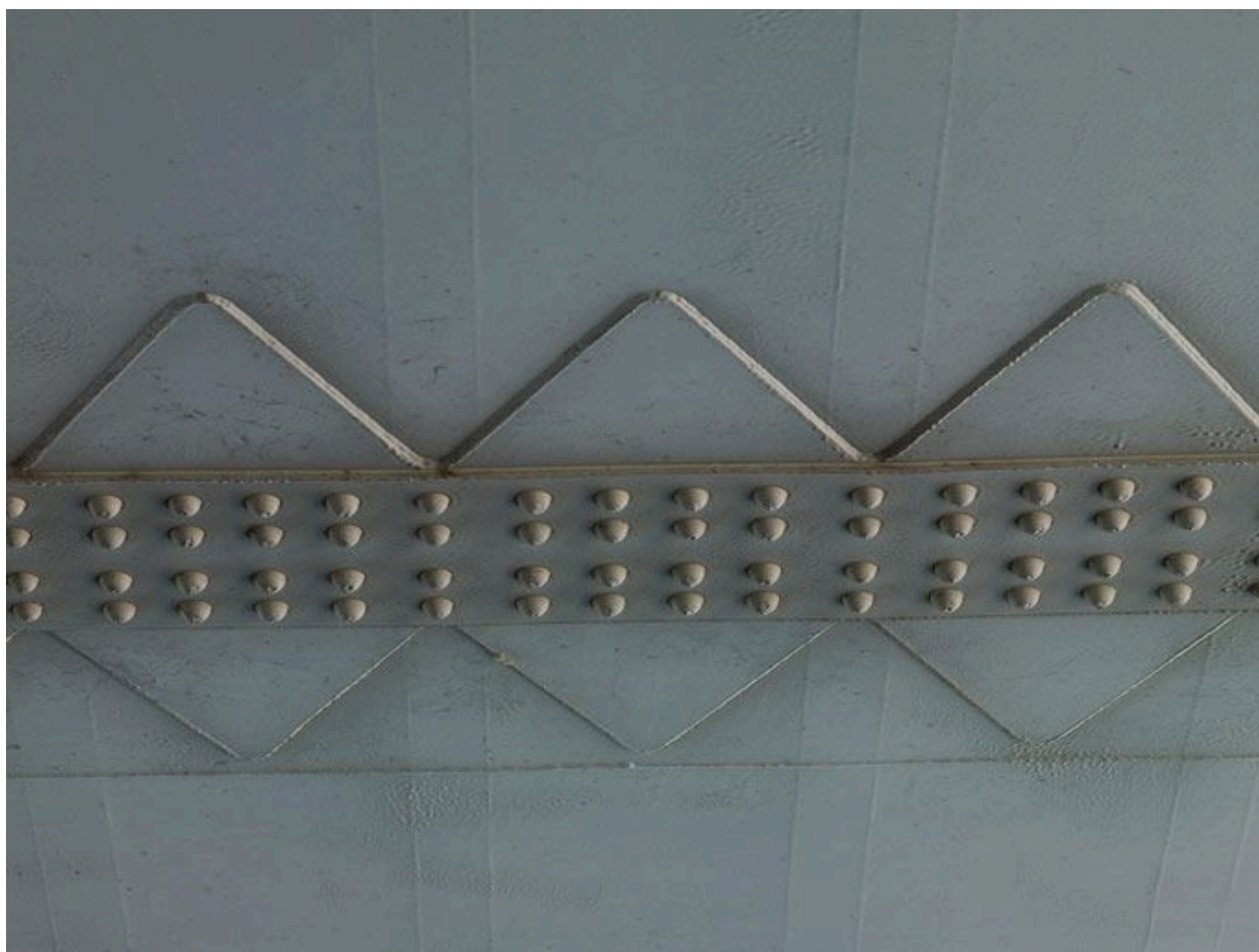
Détail de l'assemblage du tablier du pont
