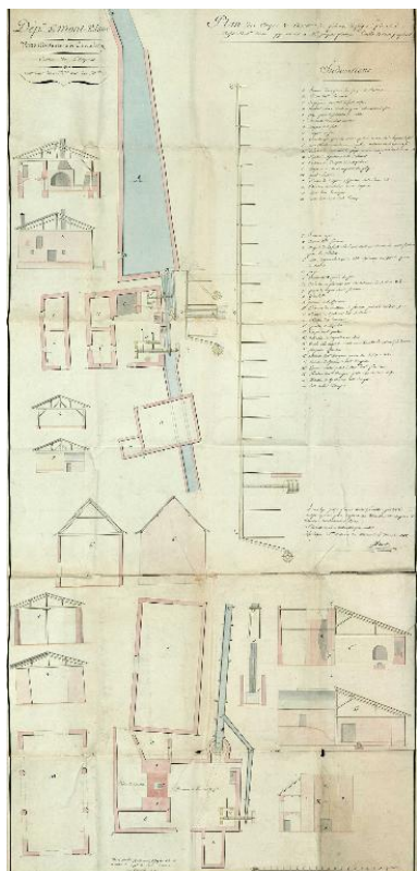
Plan de la fonderie et des forges de Sainte Hélène, 1812 (FR.AD073, 1Fi100). IVR84_20167302601NUCA
