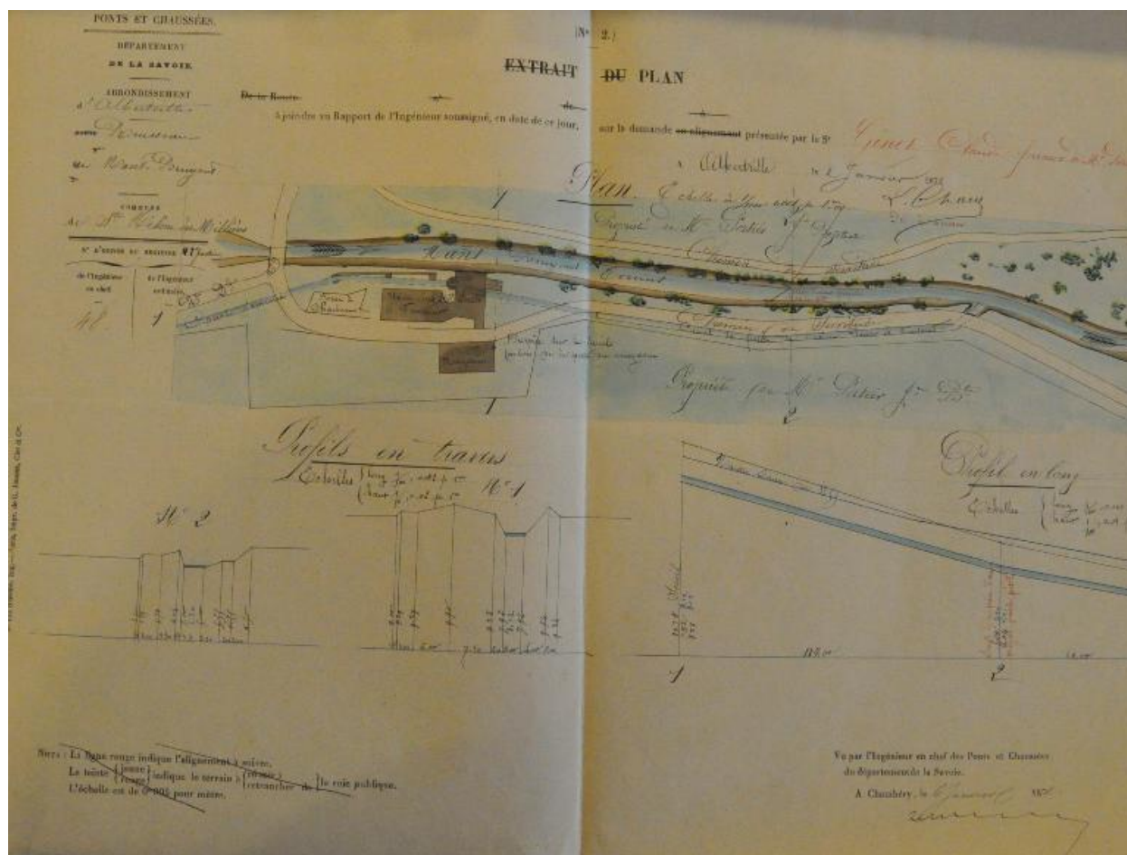
Plan accompagnant la demande de remise en activité du haut-fourneau, 1869 (FR.AD073, 82S30).
