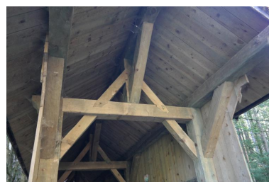
Pont couvert de Bellevaux, détail de la charpente Phot. Pascale Renard IVR84_20207401524NUCA
