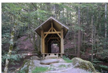
Pont couvert de Bellevaux, vue depuis la rive gauche Phot. Pascale Renard IVR84_20207401523NUCA
