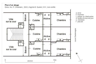
Plan des appartements du 4e étage, d'après B. Guérin, 1911 Dess. Paul Cherblanc, Autr. Guérin B. (architecte) IVR82_20036903351NUD
