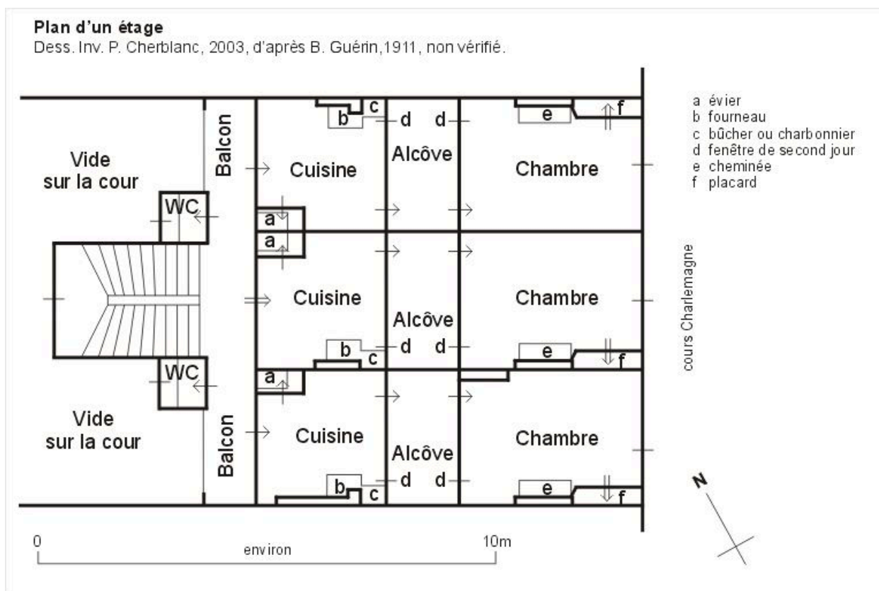
Plan des appartements du 4e étage, d'après B. Guérin, 1911
