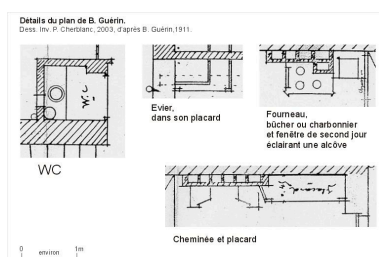
Plan du 4e étage. Détails d'aménagement, d'après B. Guérin, 1911 Dess. Paul Cherblanc, Autr. Guérin B. (architecte) IVR82_20036903352NUD
