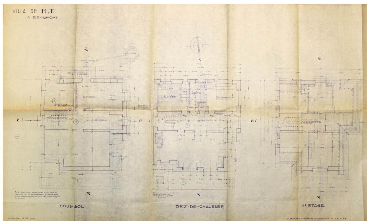
Beaumont, la maison D., plans des niveaux, 23 mars 1948, Jean Bosser architecte (Archives départementales du Puy-de-Dôme, Fonds de la Direction départementale de l'Équipement, 1611 W 37, PC n° D 686).
