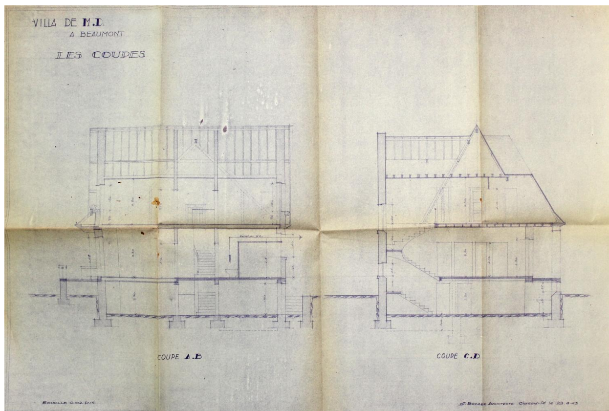
Beaumont, la maison D., les coupes, 23 mars 1948, Jean Bosser architecte (Archives départementales du Puy-de-Dôme, Fonds de la Direction départementale de l'Équipement, 1611 W 37, PC n° D 686).
