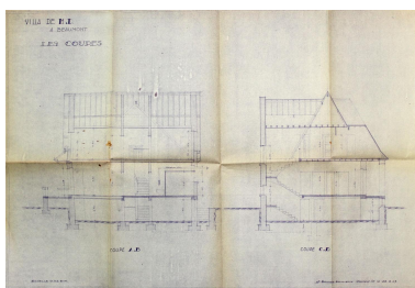
Beaumont, la maison D., les coupes, 23 mars 1948, Jean Bosser architecte (Archives départementales du Puy-de-Dôme, Fonds de la Direction départementale de l'Équipement, 1611 W 37, PC n° D 686). Repro. Christophe Laurent, Autr. Jean Bosser IVR84_20216302553NUCA
