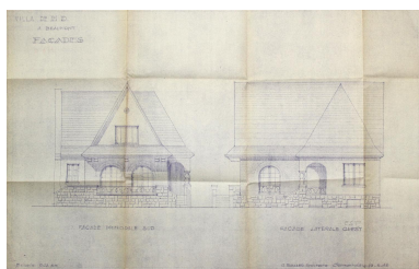
Beaumont, la maison D., façade principale sud et façade latérale est, 23 mars 1948, Jean Bosser architecte (Archives départementales du Puy-de-Dôme, Fonds de la Direction départementale de l'Équipement, 1611 W 37, PC n° D 686). Repro. Christophe Laurent, Autr. Jean Bosser IVR84_20216302552NUCA
