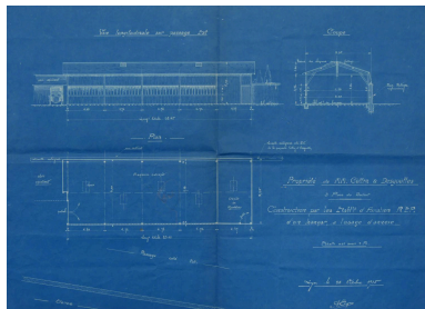
Hangar à usage d'annexe Cottin-Desgouttes 1915 (ACL : 314W564-165) Phot. Nadine Halitim-Dubois IVR84_20246900106NUCA
