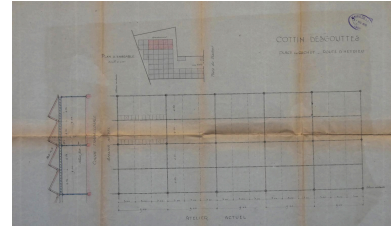
Plan d'ensemble 1912, usine Cottin Desgoutte (ACL : 314W469-804) Phot. Nadine Halitim-Dubois IVR84_20246900081NUCA
