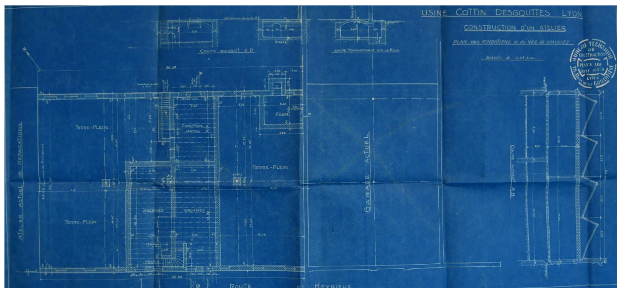
Plan des fondations et du rez-de-chaussée 1918 (AC Lyon314W/601)
