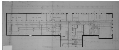
Construction d'un service de polyomélitiques [bâtiment W], par J. Favier et R. Genin, 1959-1960, feuille 7A, Sous-sol. Aile A Phot. Didier Gourbin IVR82_20056900346NUC
