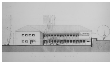
Construction d'un service de polyomélitiques [bâtiment W], par J. Favier et R. Genin, 1959-1960, feuille 10, façade ouest Phot. Didier Gourbin IVR82_20056900350NUC
