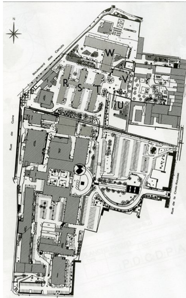
Plan-masse de l'hôpital avec localisation des principaux bâtiments à démolir, extrait du permis de démolir par l'atelier Ch. de Portzamparc, 25 mai 2004 Phot. Bernard Ducouret IVR82_20056901079NUC
