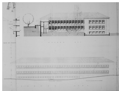
Construction d'un service de polyomélitiques [bâtiment W], par J. Favier et R. Genin, 1959-1960, feuille 10, façades est et nord Phot. Didier Gourbin IVR82_20056900348NUC
