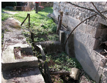
Conduit d'amenée de l'eau du bief sur le lieu où se trouvait la roue à aube du moulin. Phot. Thierry Monnet IVR82_20144200194NUCA
