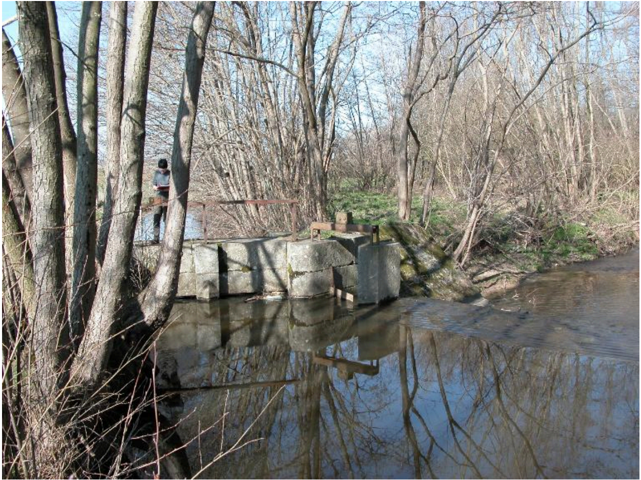
Vue d'ensemble amont de la prise d'eau en pierre de taille.
