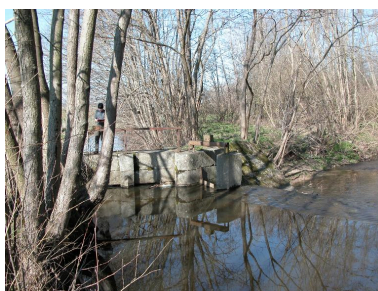
Vue d'ensemble amont de la prise d'eau en pierre de taille. Phot. Thierry Monnet IVR82_20144200186NUCA
