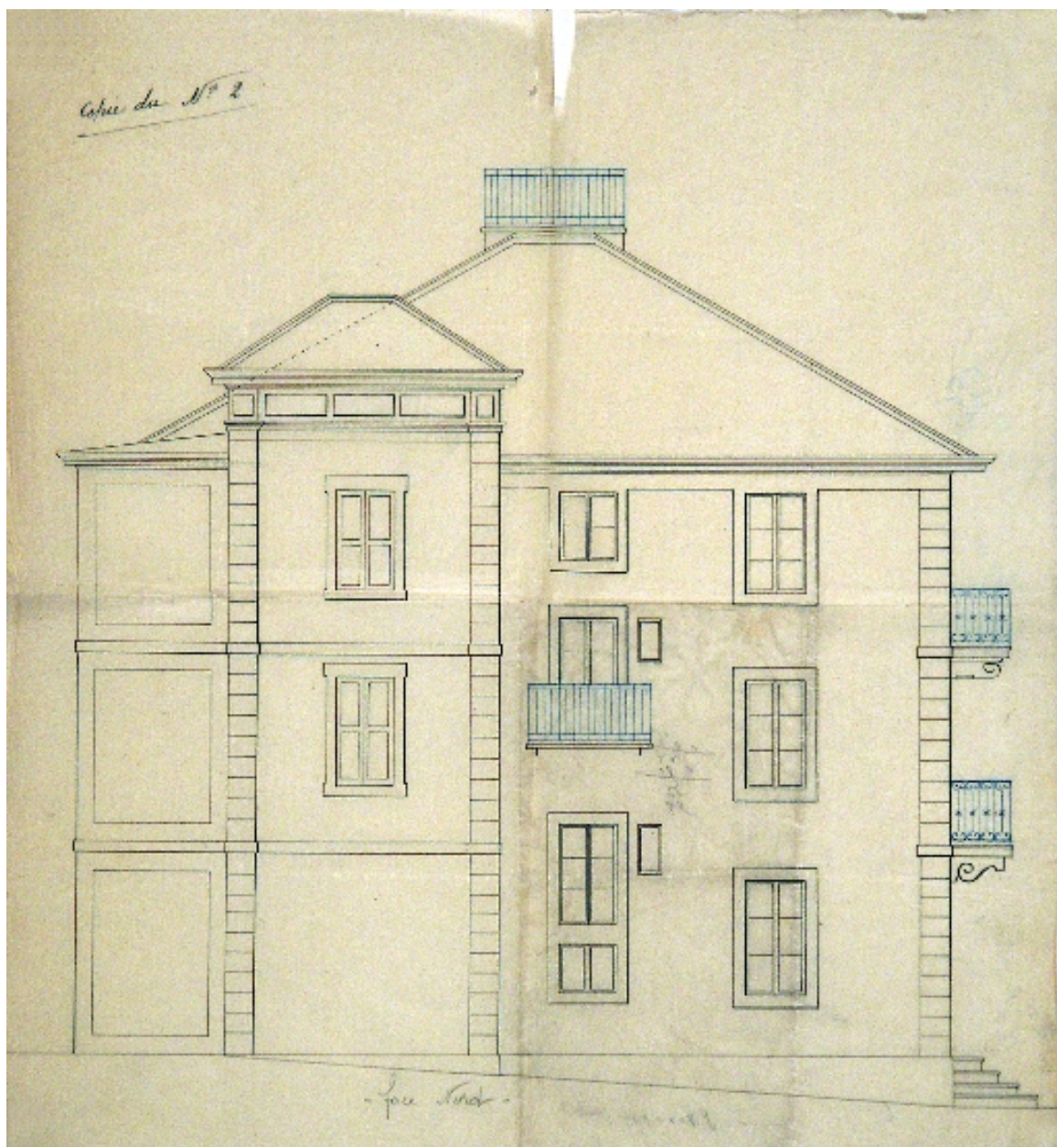
Elévation nord de la villa
