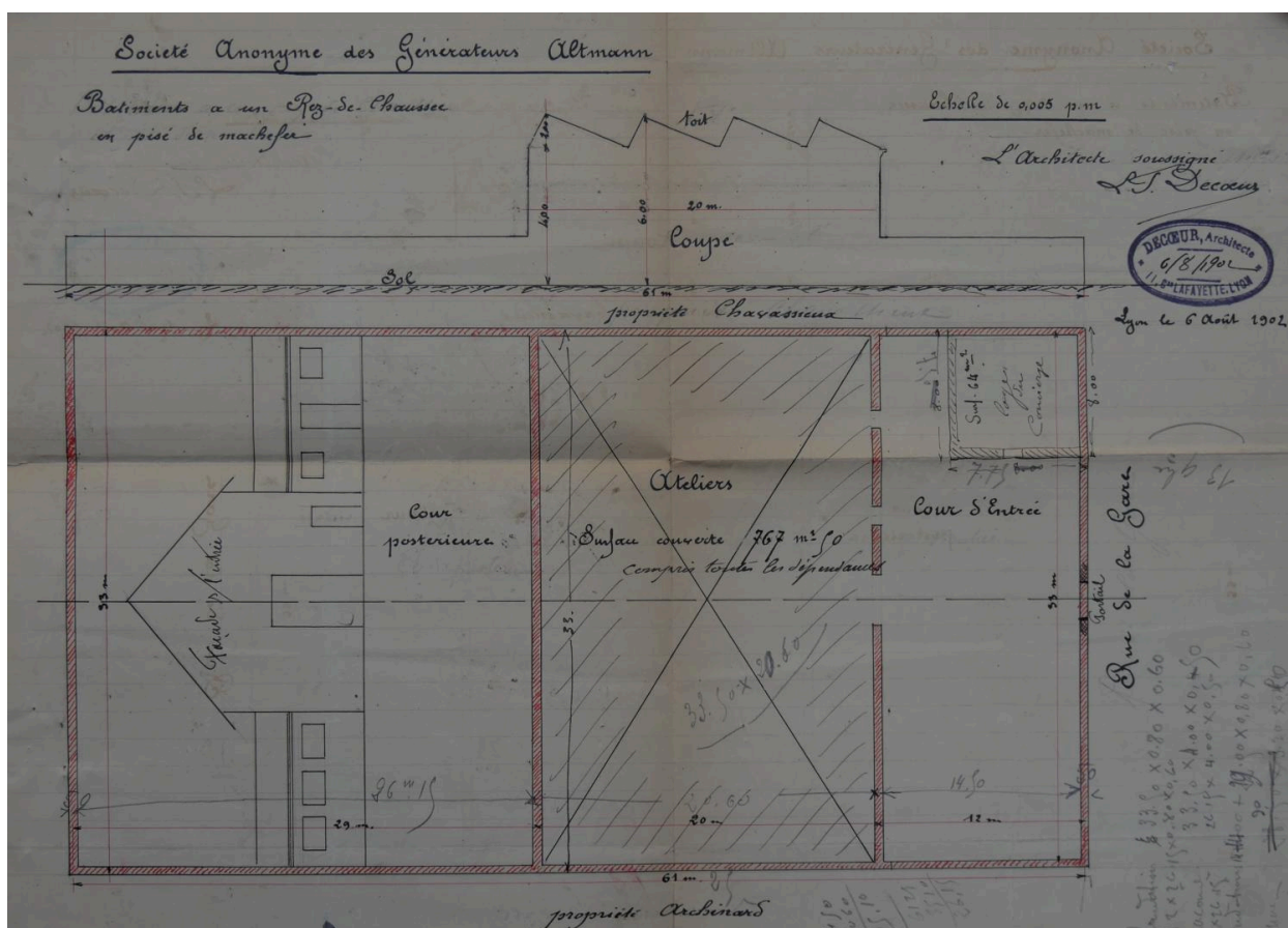
Plan masse bâtiments rez-de-chaussée usine Générateurs Altmann 1902 (ACL : 314W184, 418)
