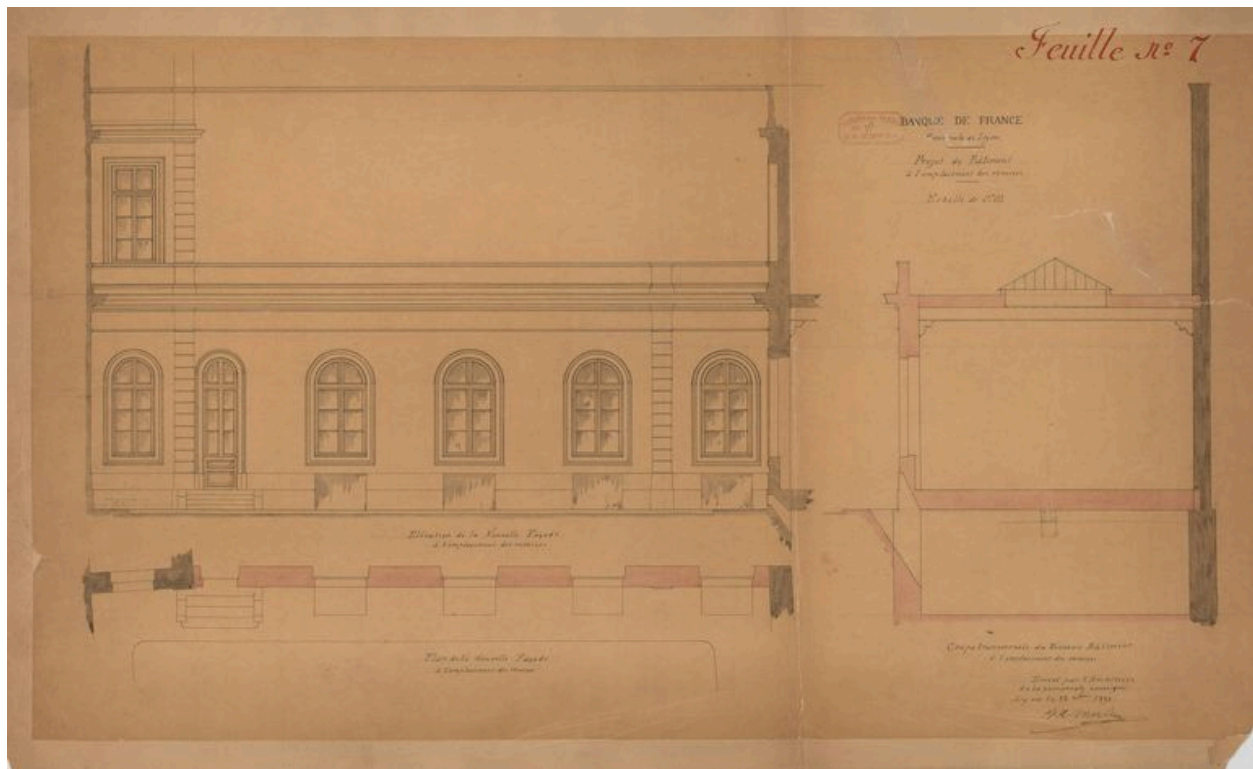
Élévation et coupe de l'annexe construite dans la cour (1891) (Banque de France, service du Patrimoine Historique et Artistique, non coté, dessin de Jean-Claude Merlin).
