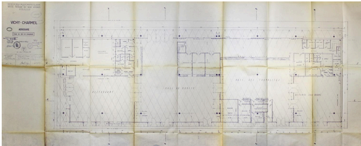
Plan du rez-de-chaussée de l'aérogare de Vichy-Charmeil, février 1955, Service technique des bases aériennes (Archives municipales de Vichy).
