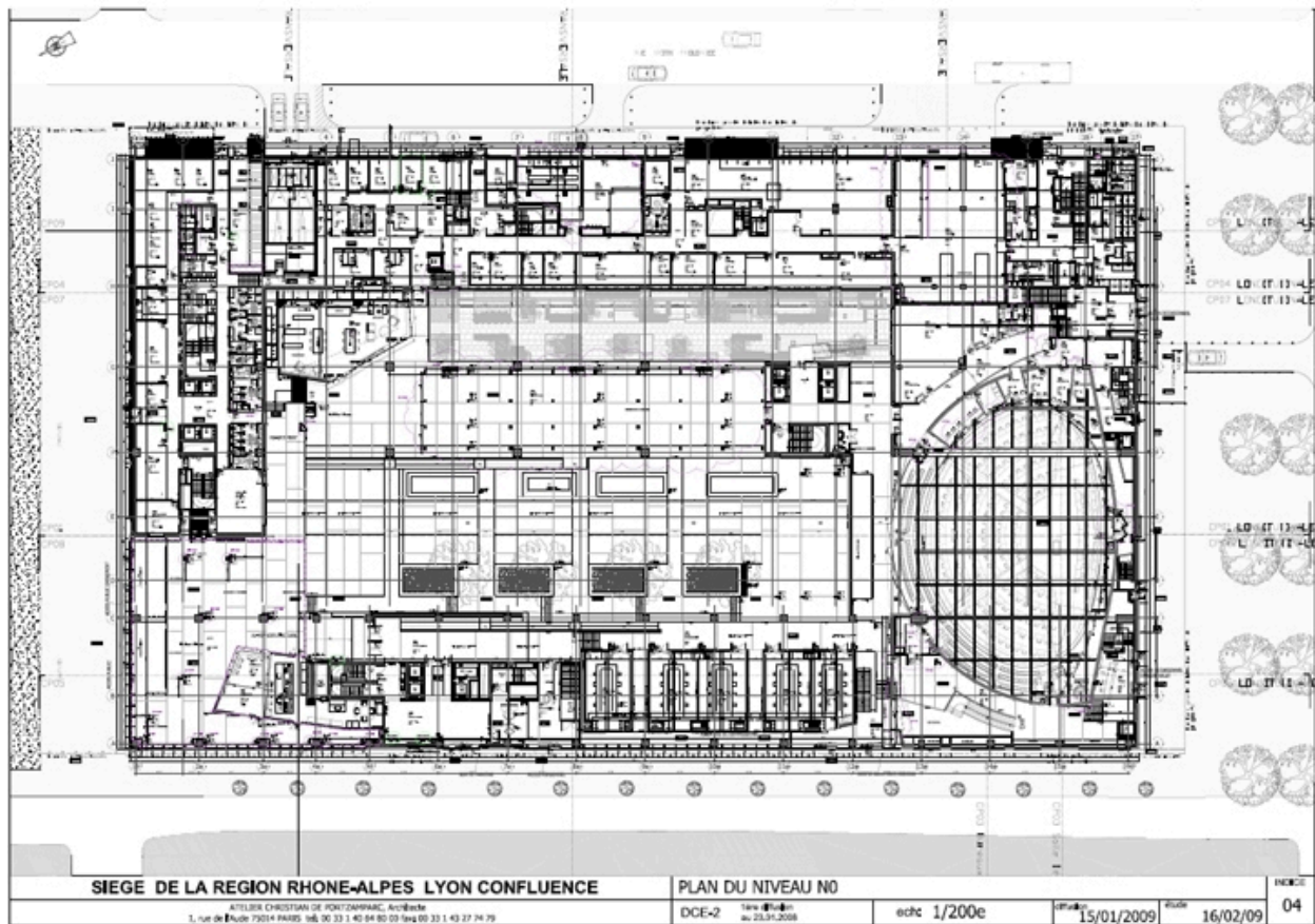
Plan du niveau N0 (rez-de-chaussée) : siège de la Région Rhône-Alpes Lyon Confluence
