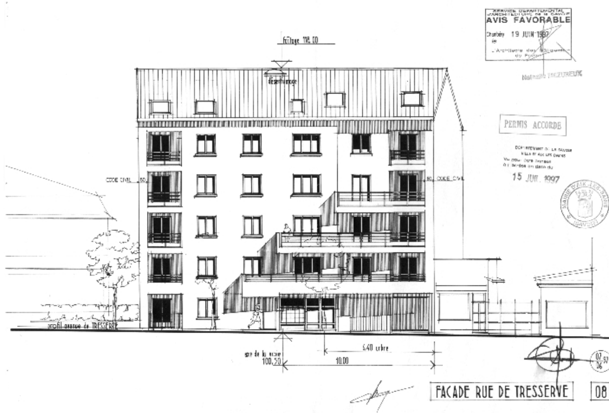
Elévation principale
