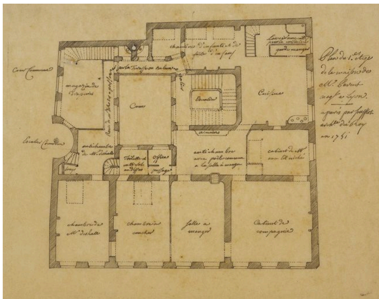
Plan du 1er étage de la maison de M. Parent négociant à Lyon, copie d'après Soufflot, 1751
