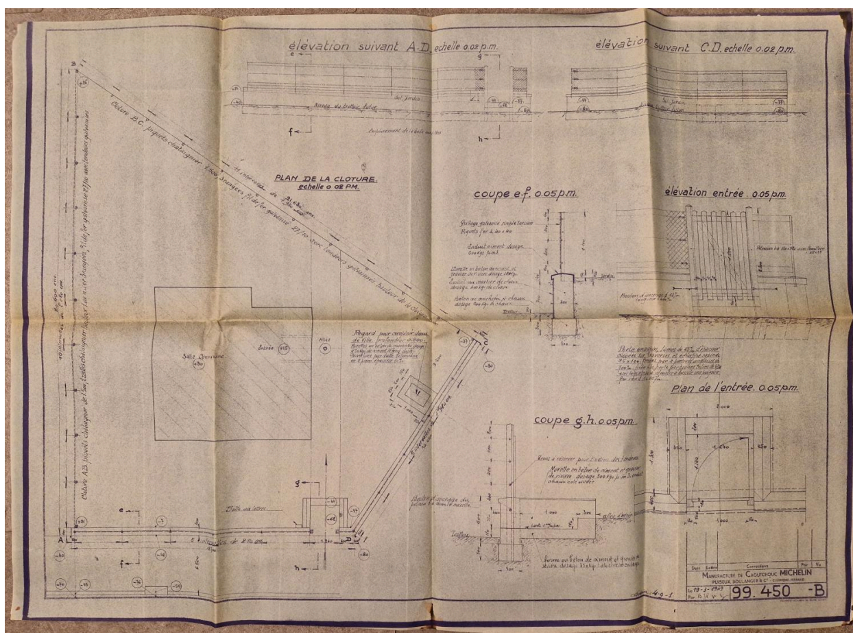
Cité Barbier-Daubrée : plans, coupes et élévations du mur de clôture de la première maison prototype. Tirage sur papier, échelles 0,002 et 0,005 m/m, s.n., 19/03/1949. Archives municipales de Clermont-Ferrand, cote 28 A 214.
