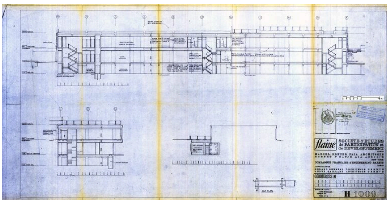
Commerces H. Coupes longitudinales et transversales. Marcel Breuer, Robert F. Gatje, 13 décembre 1962 (AC Arâches-la-Frasse)
