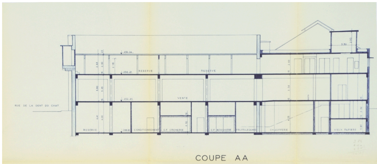
Coupe longitudinale
